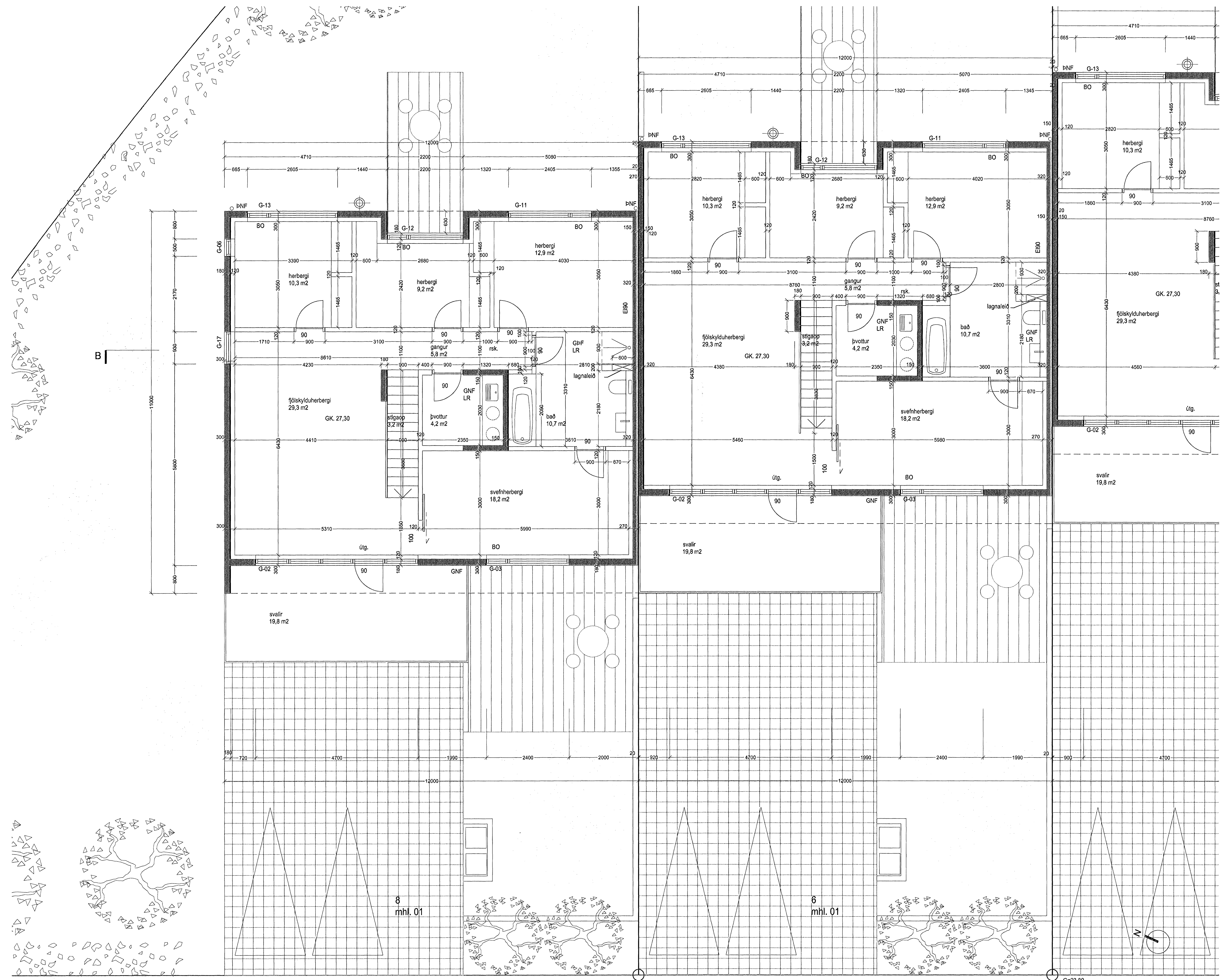
GRUNNMYND 2. HÆÐ MKV. 1:50
