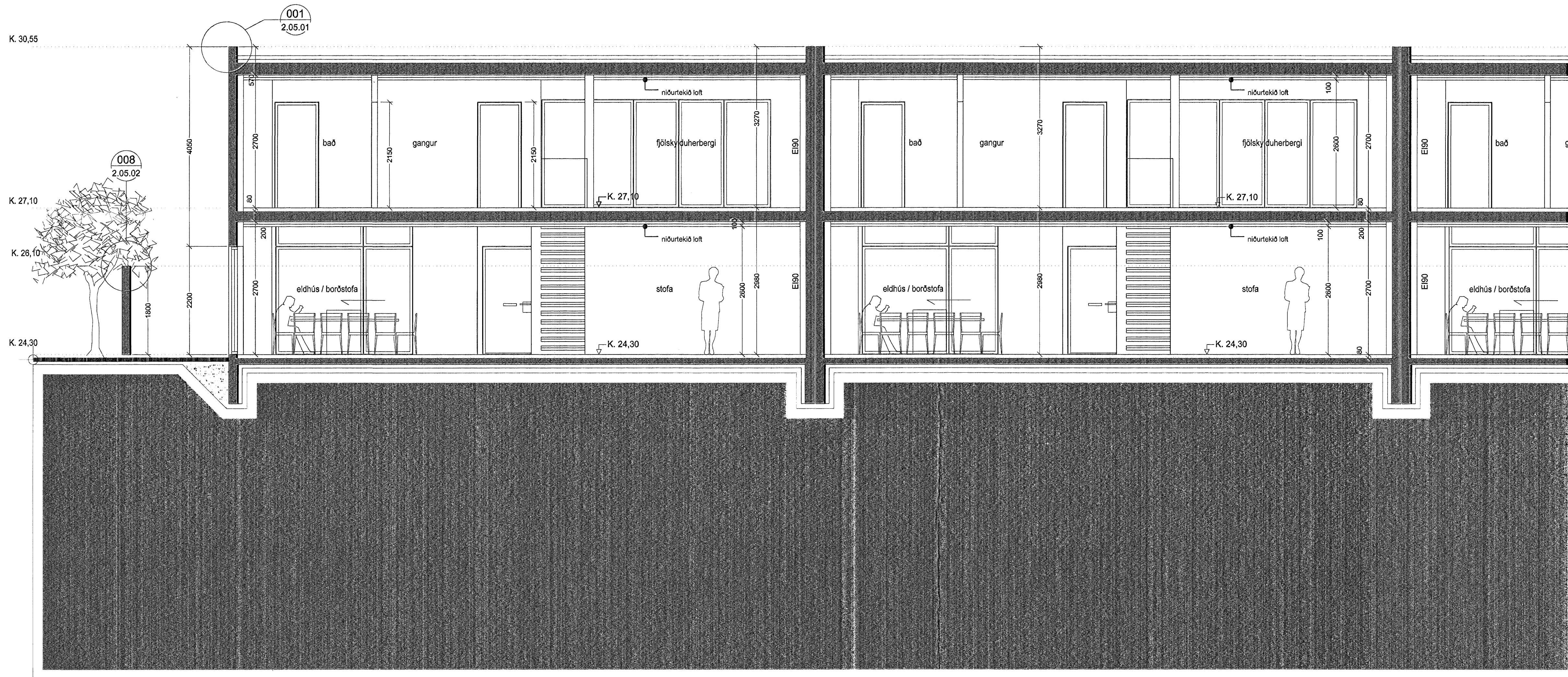
SNID A-A MKV. 1:50
