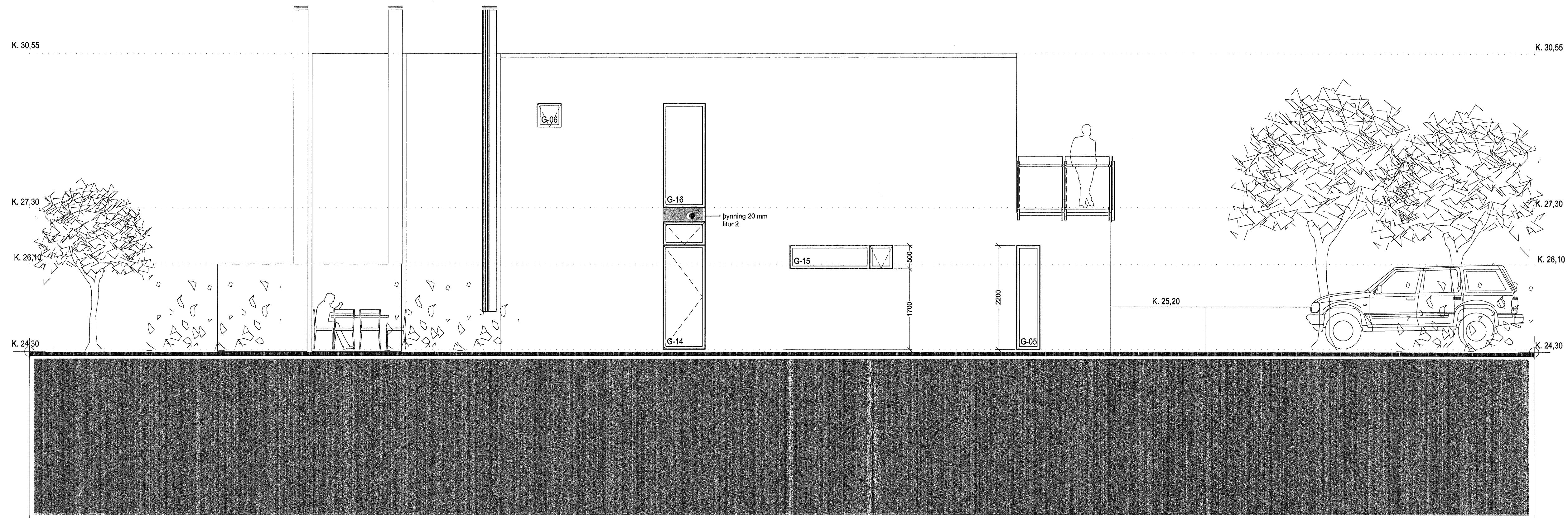
ÚTLIT TIL NORÐURS, KLUKKUVELLIR 8 MKV. 1:50
