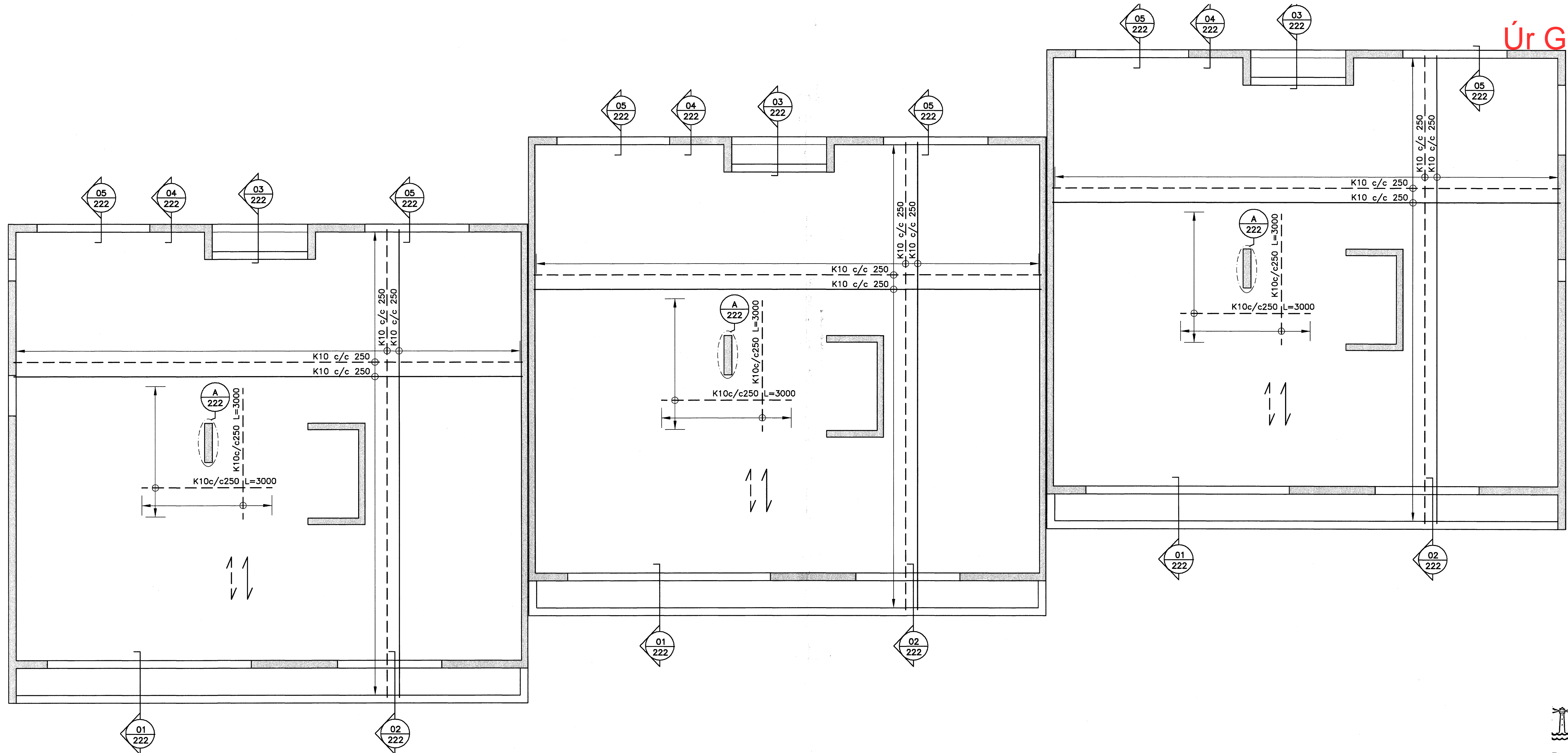
ÞAKPLATA, GRUNNMYND, 1:50
