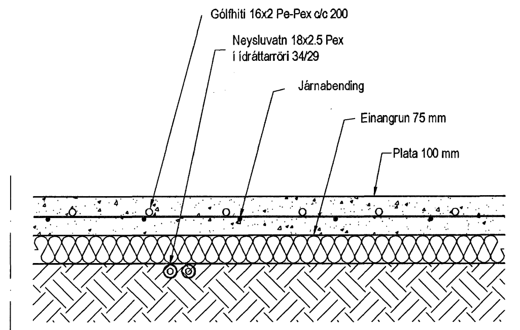
Hita- og vatnslagnir, Sníð í botnþötu, 1:10
