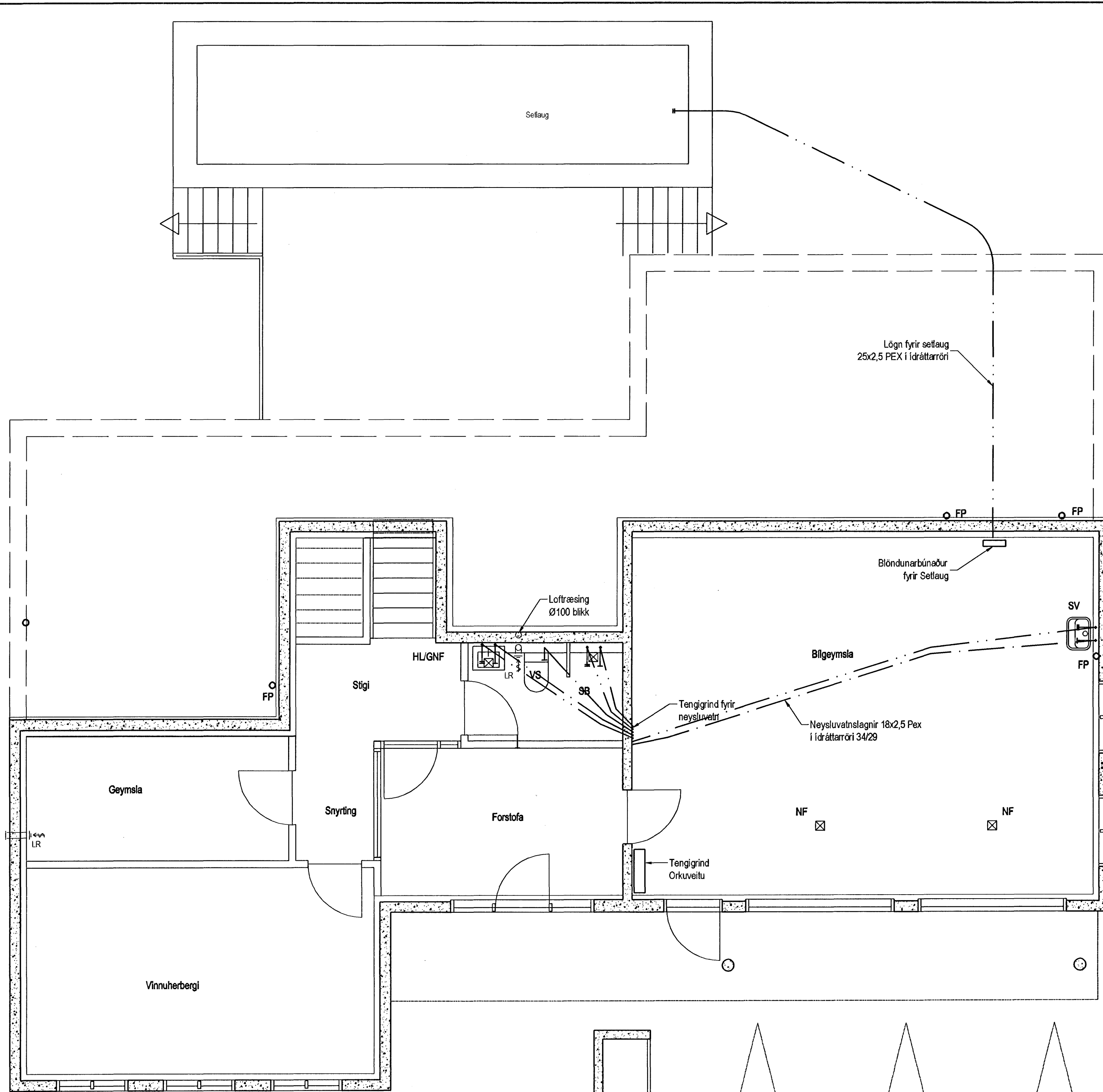
Neysluvatnslagnir 1. hæð, 1:50
