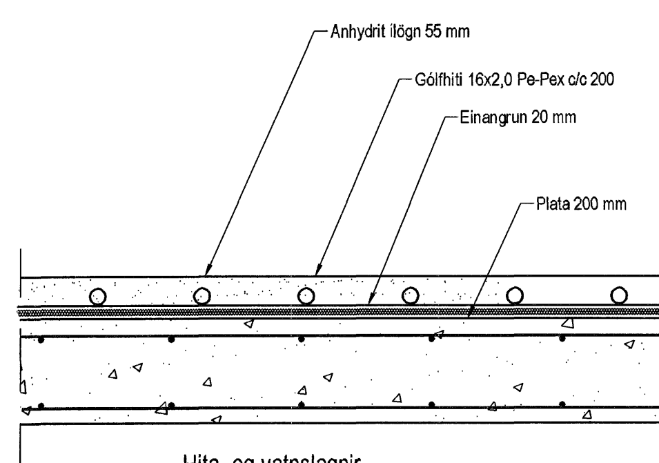
Hita- og vatnslagnir, Sníð í milliþötu, 1:10
