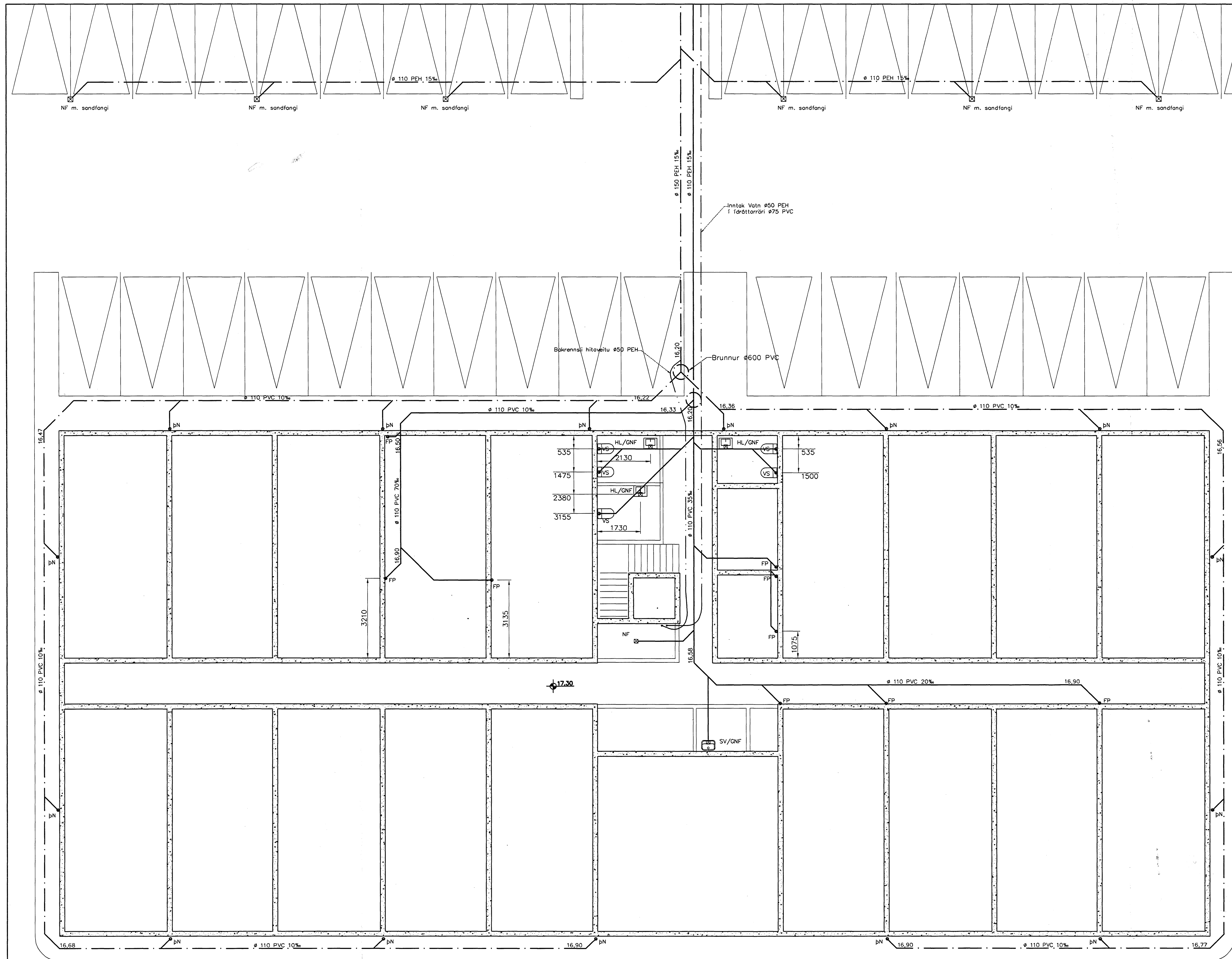
Grunnlagnir, Grunnmynd, 1:75
