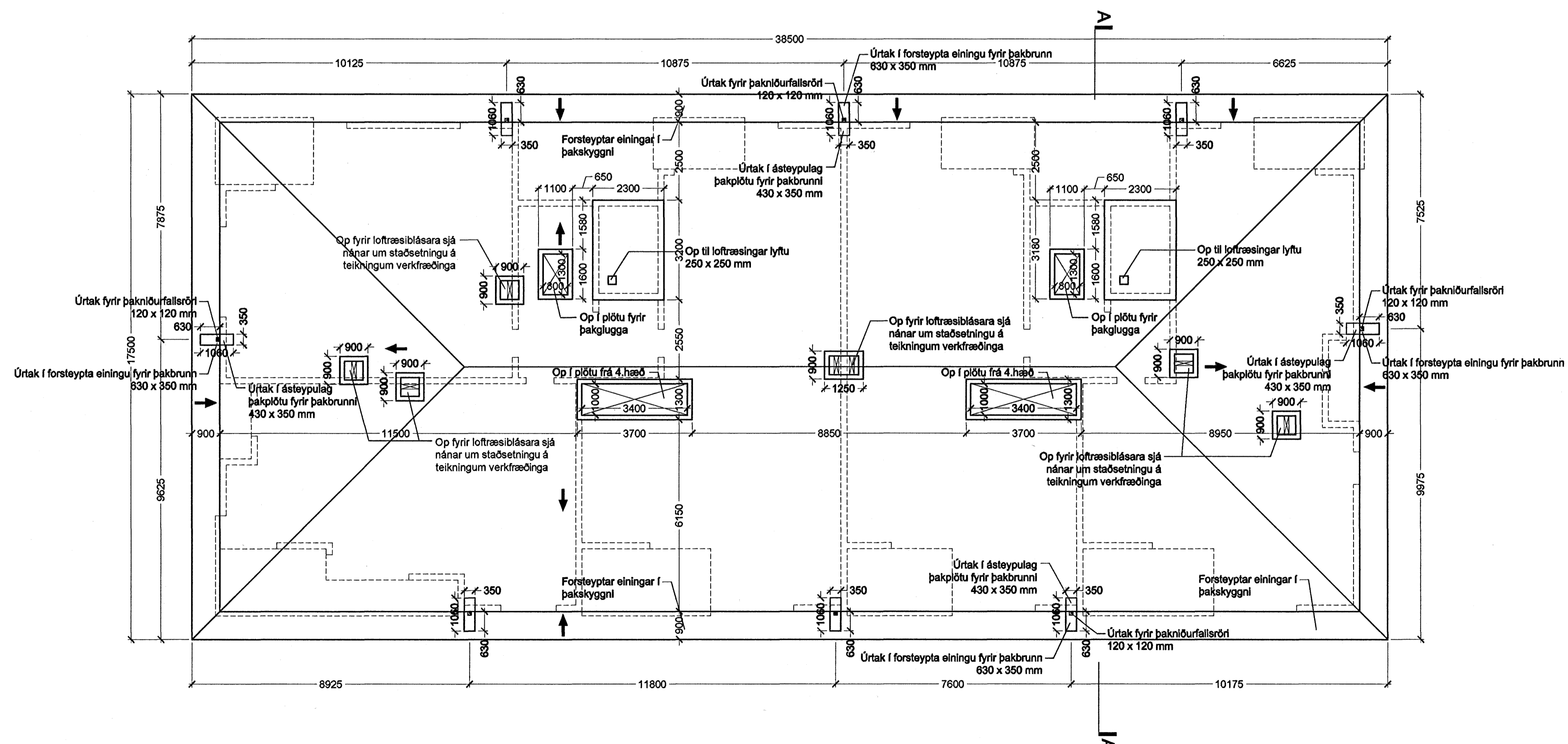
Grunnmynd þakhæðar í mkv. 1:100
