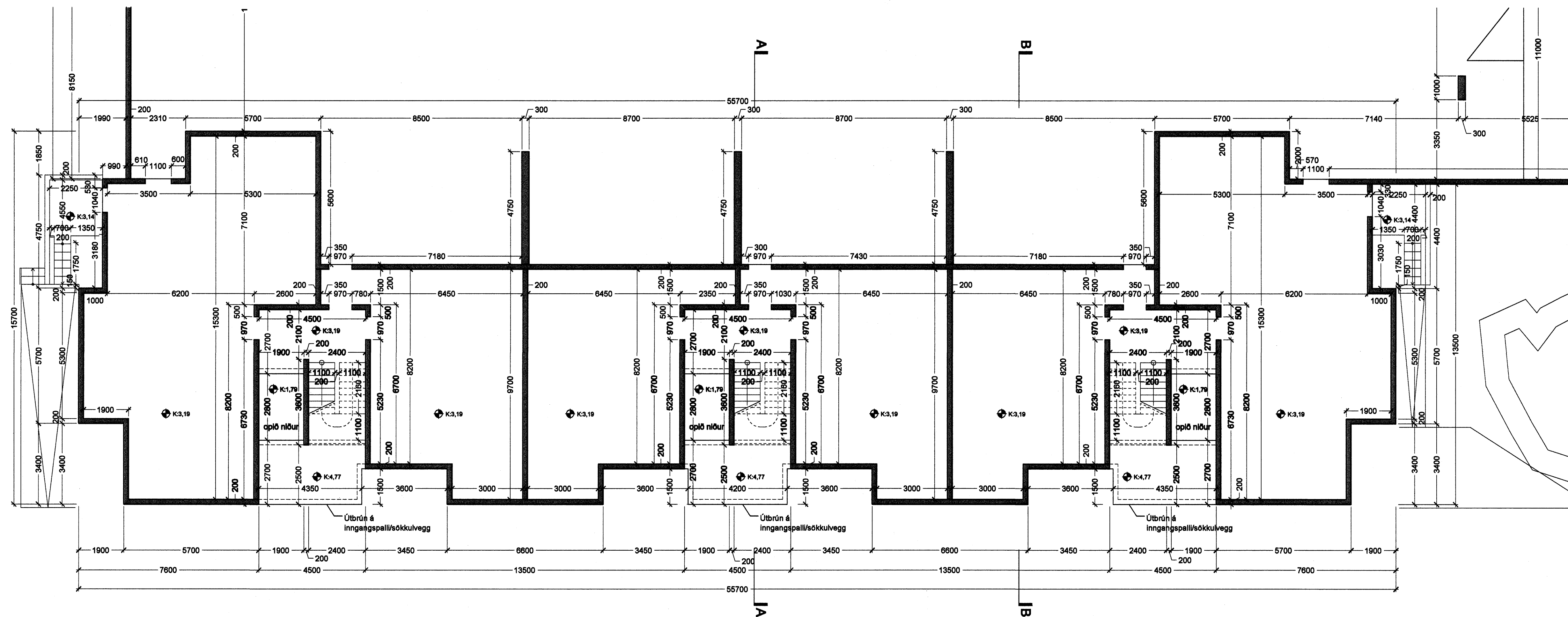
Grunnmynd kjallara í mkv. 1:100
