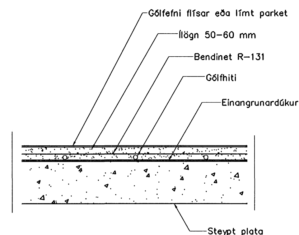
Gólfhiti snið, 1:10
