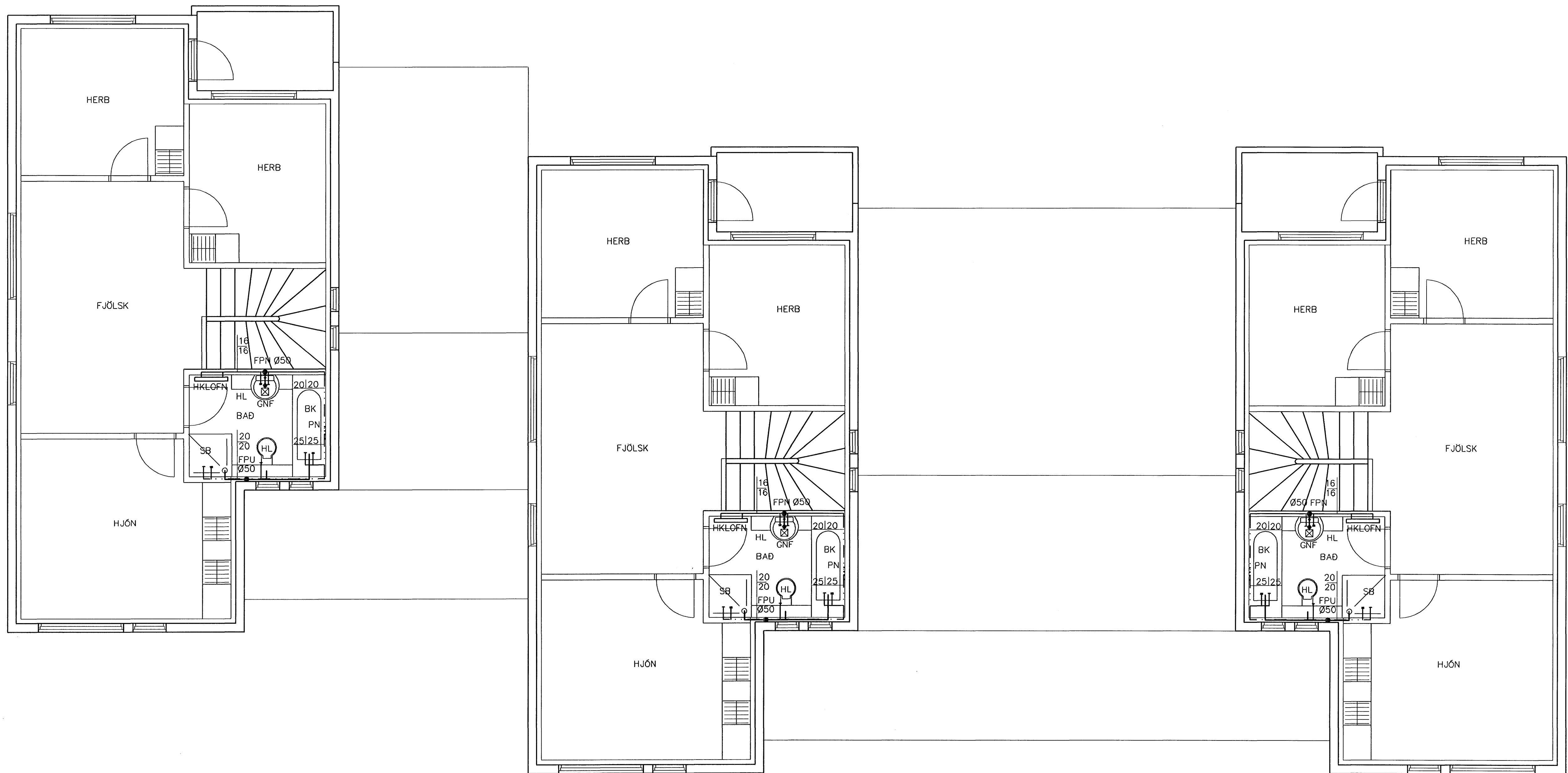
GRUNNMYND 2 HÆÐAR 1:50
