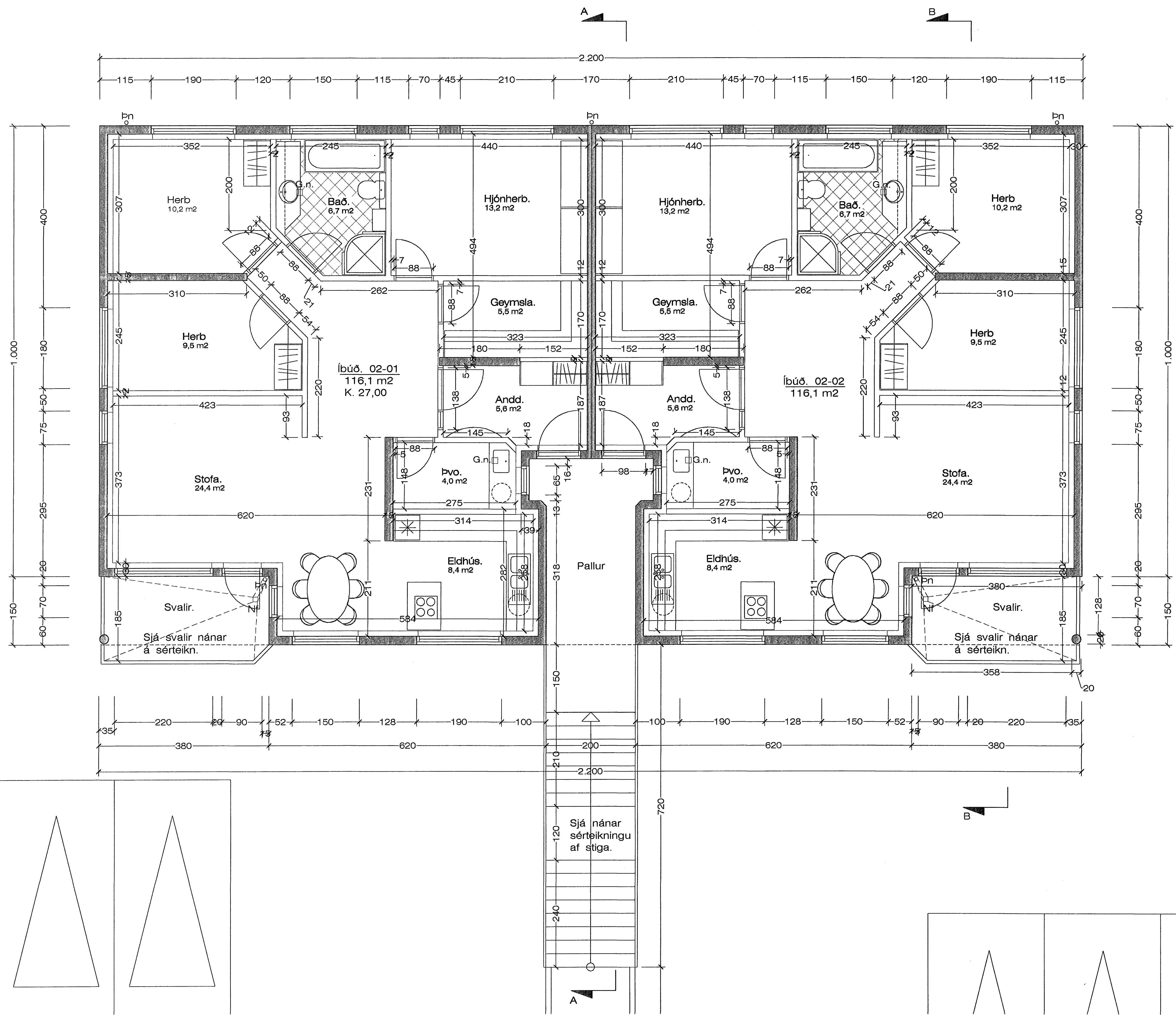
Grunnmynd 2. hæð. 1 : 50
