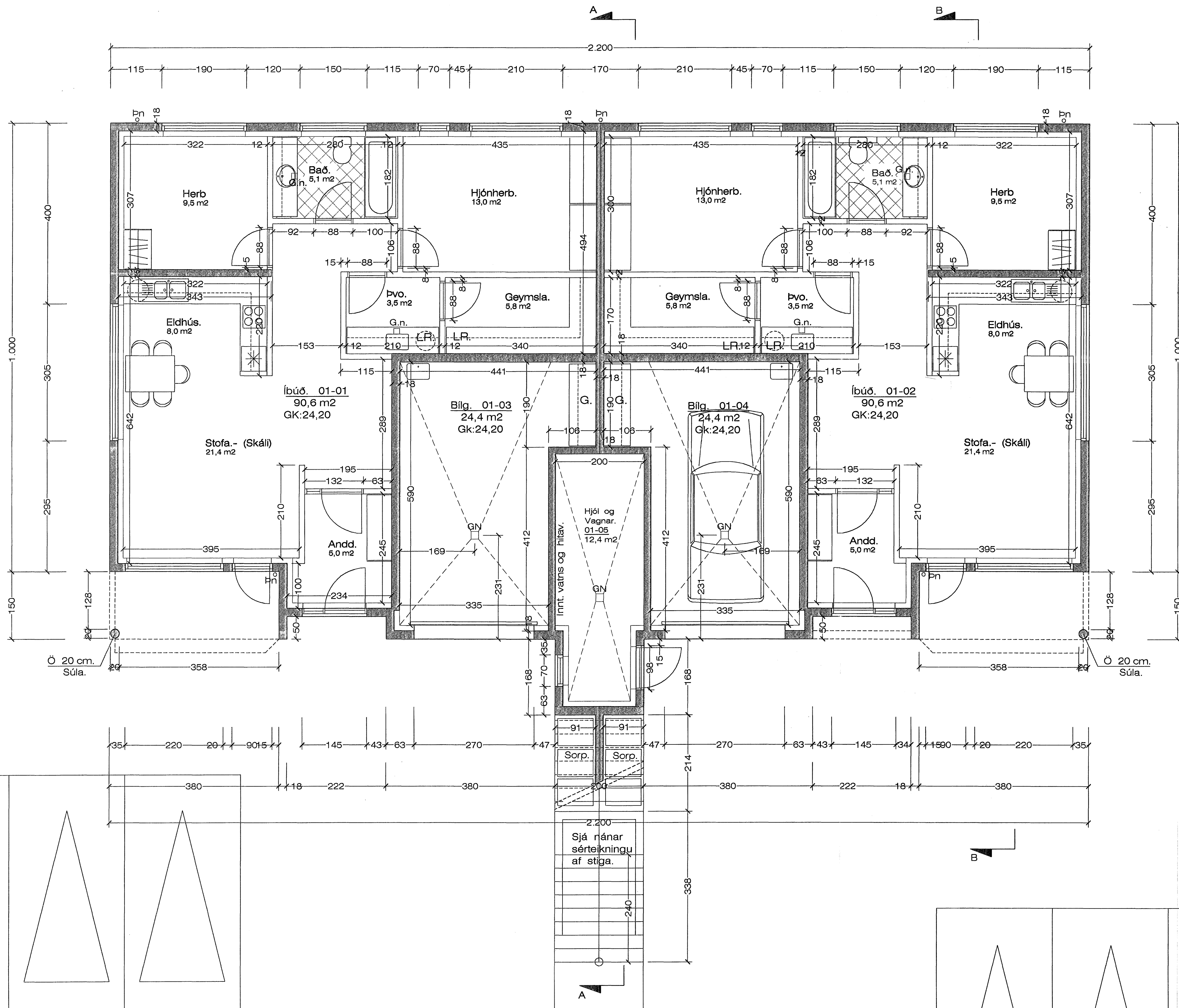
Grunnmynd 1. hæð. 1 : 50
