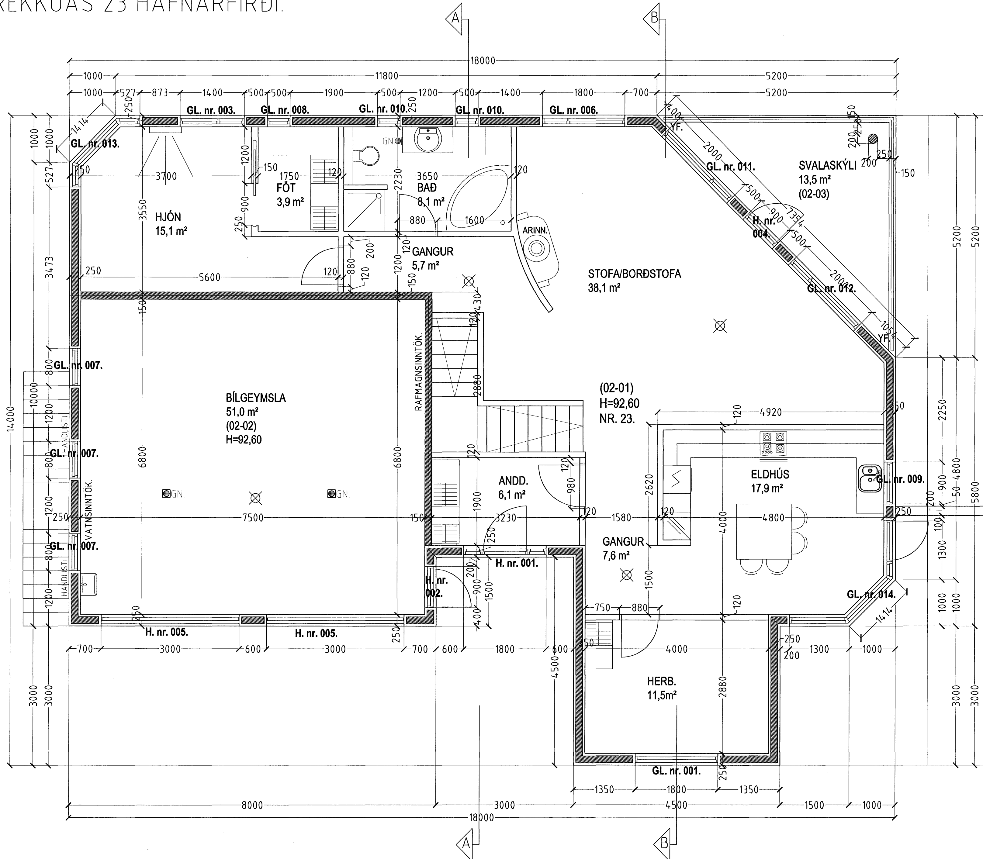
GRUNNMYND 2. HÆÐ MKV. 1:50.
