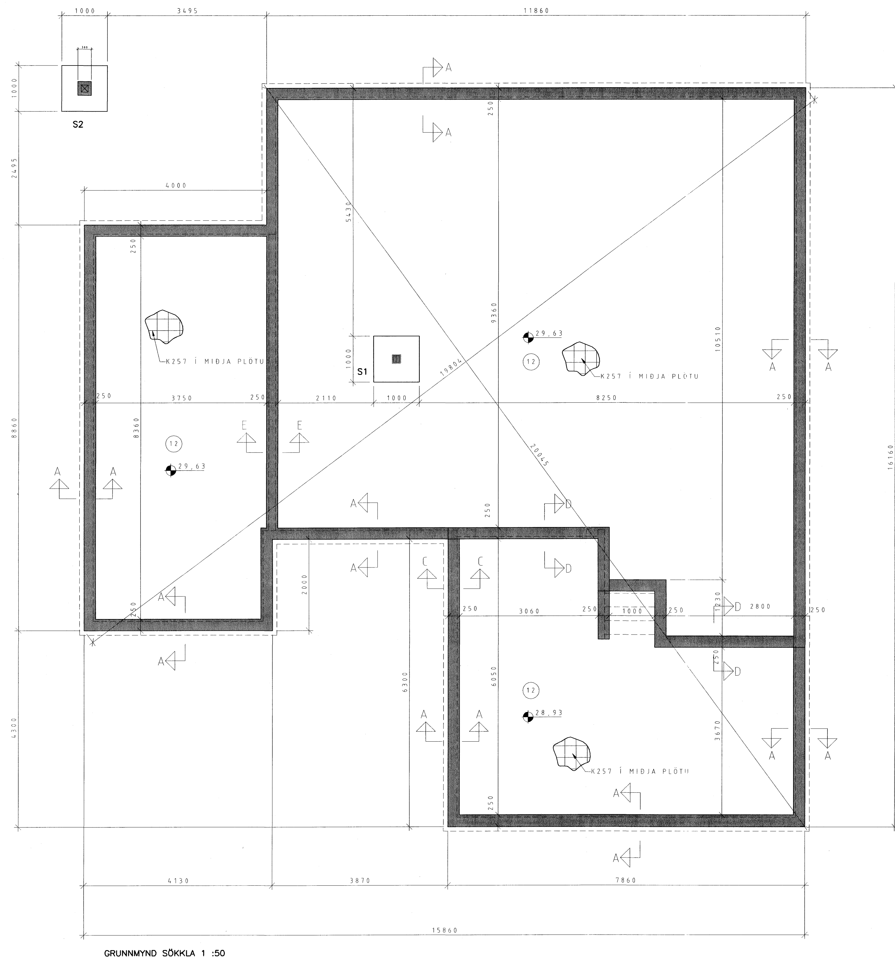
GRUNNMYND SÖKKLA 1 :50
