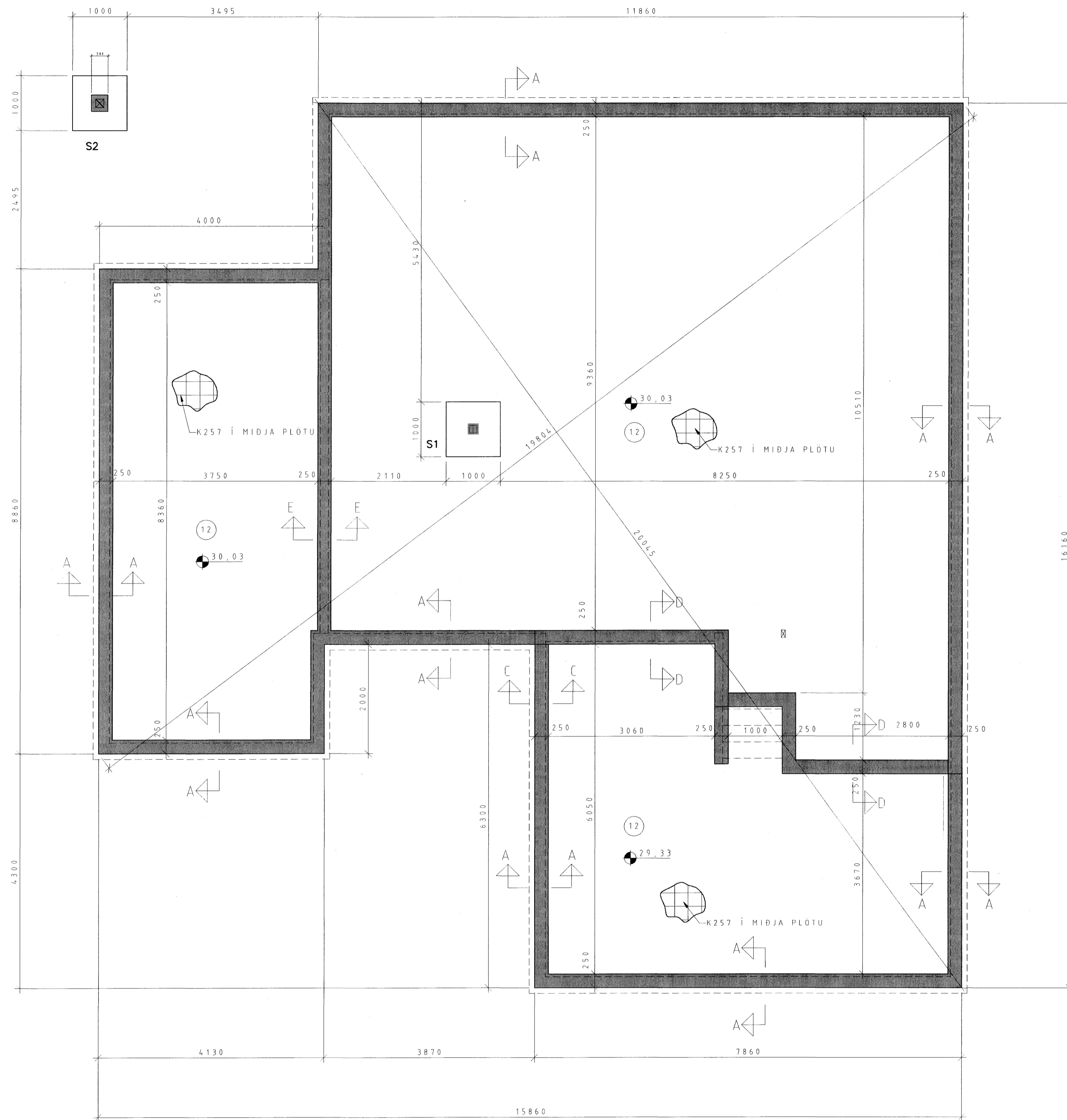
GRUNNMYND SÖKKLA 1 :50
