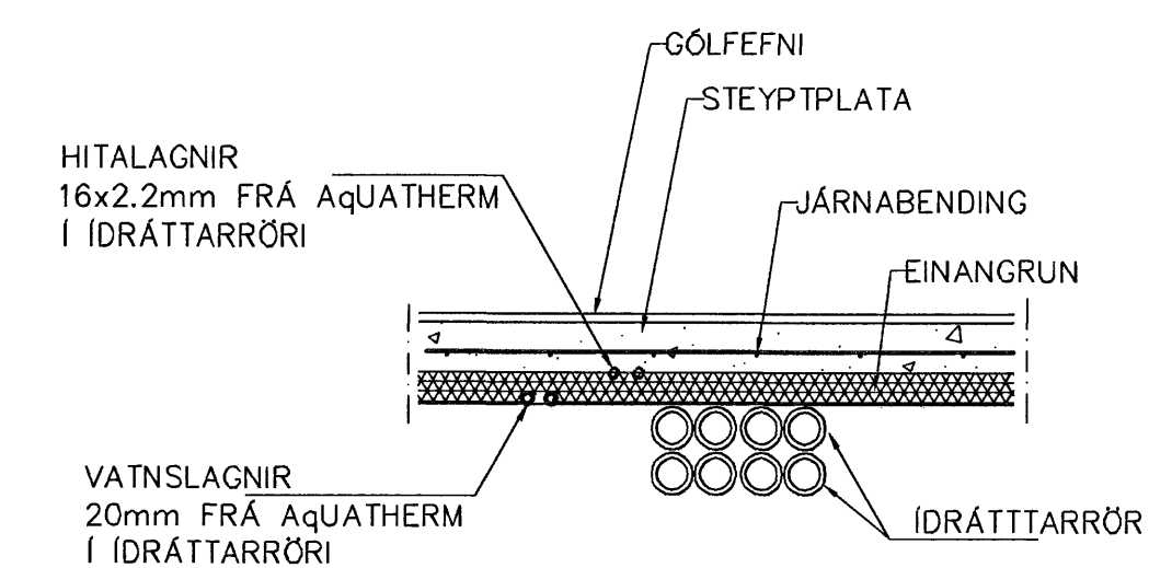
LAGNIR, SNIÐ, 1:20
