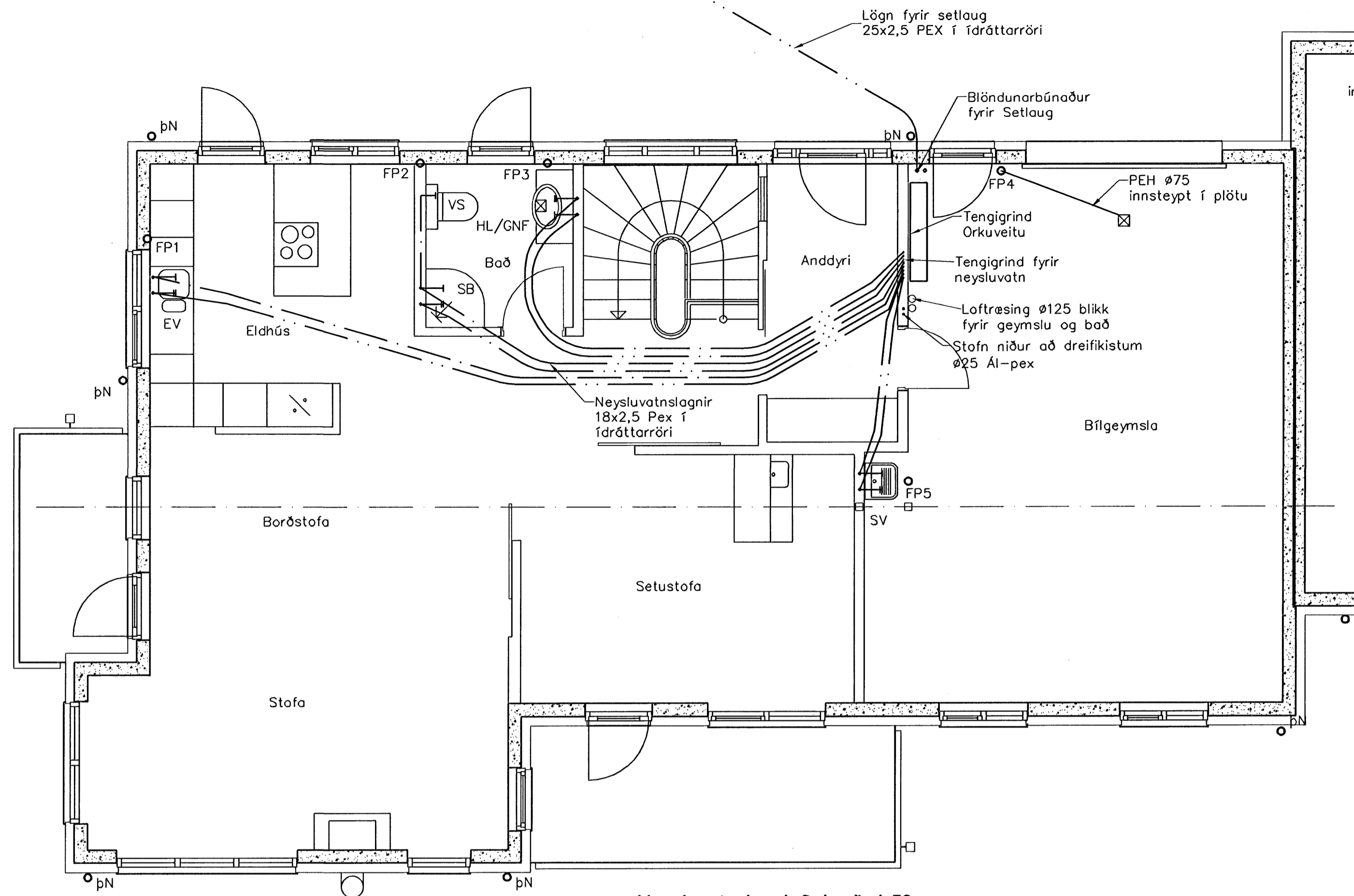
Neysluvatnslagnir 2. hæð, 1:50
