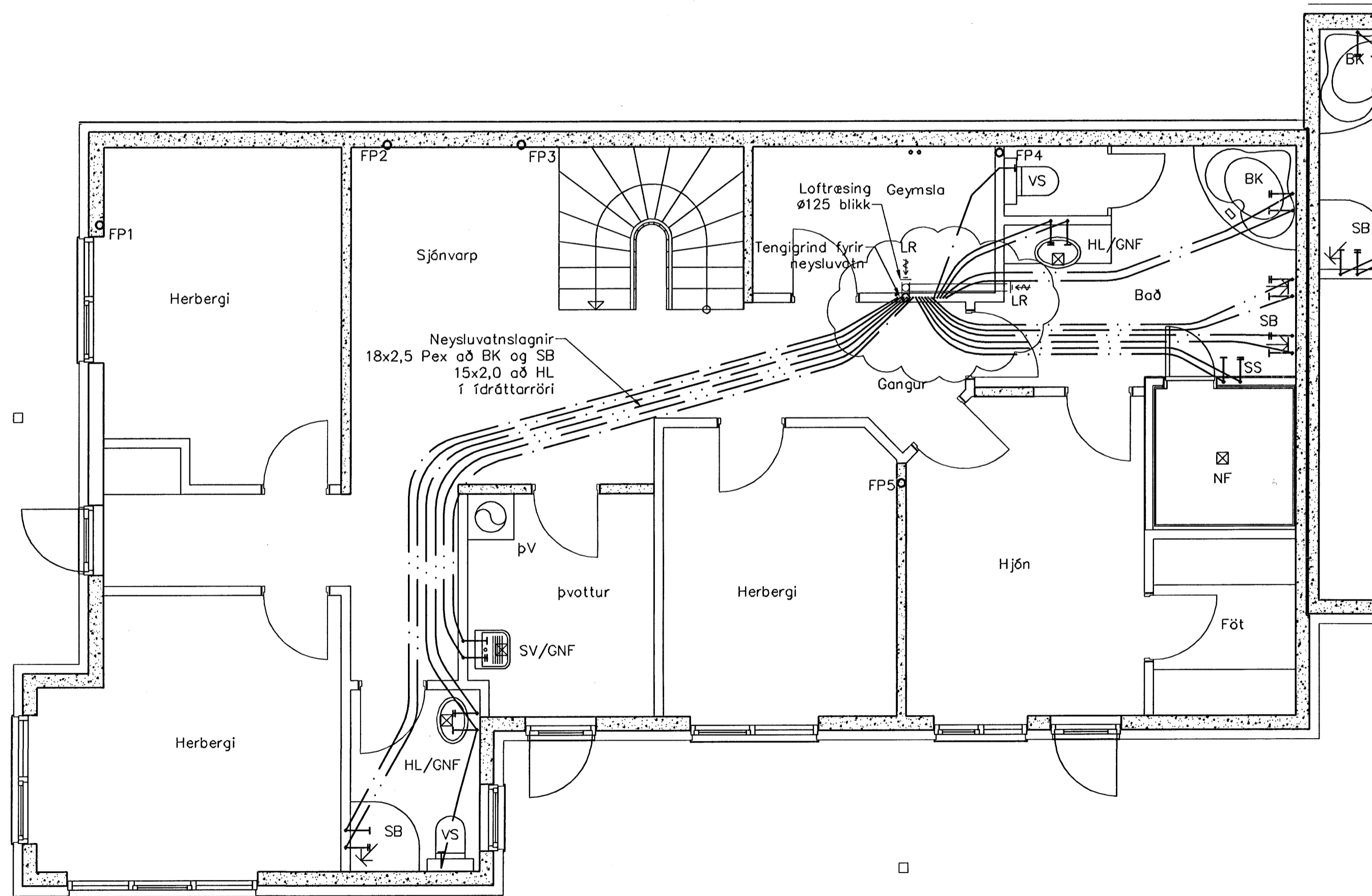
Neysluvatnslagnir 1. hæð, 1:50
