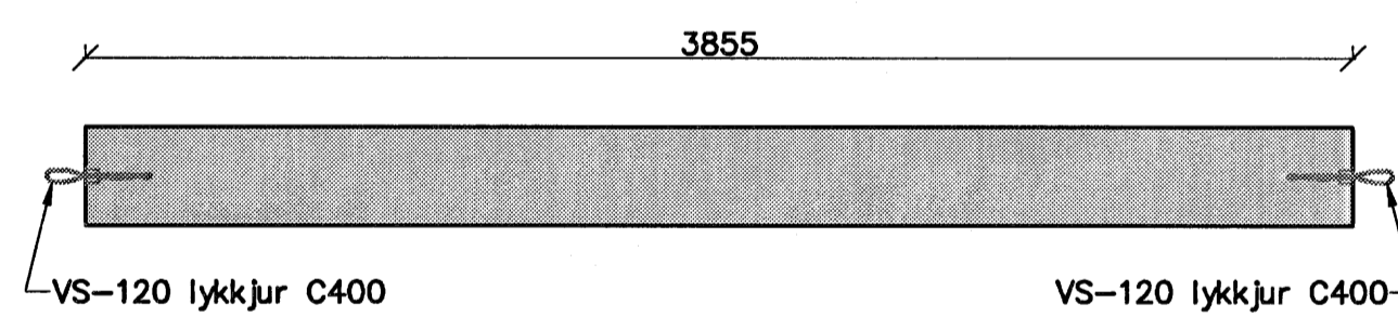
Eining M3 1:25 1stk.
