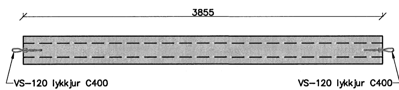
Eining M1 1:25 3stk.
