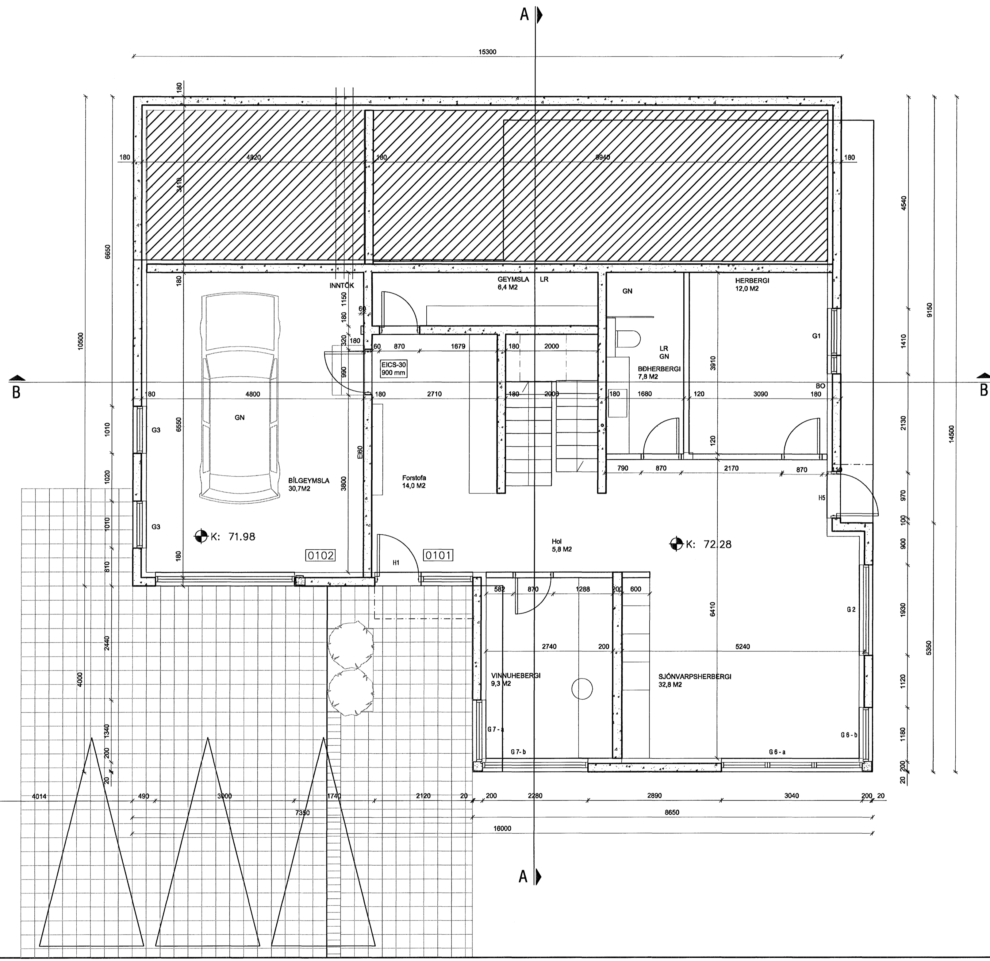
GRUNNMYND 1. HÆÐ
