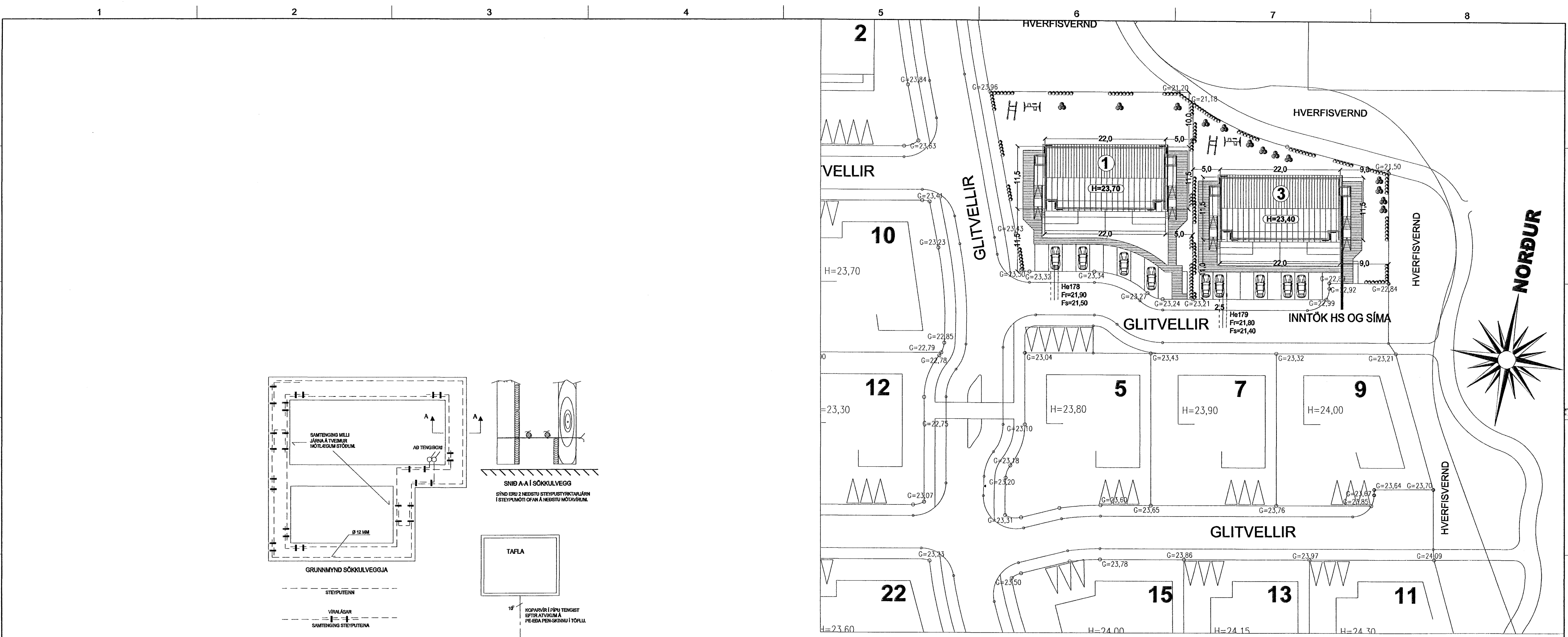
AFSTÖÐUMYND MKV. 1:500
