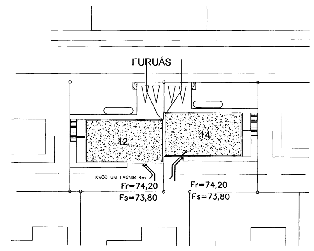
Afstöðumynd 1:500
