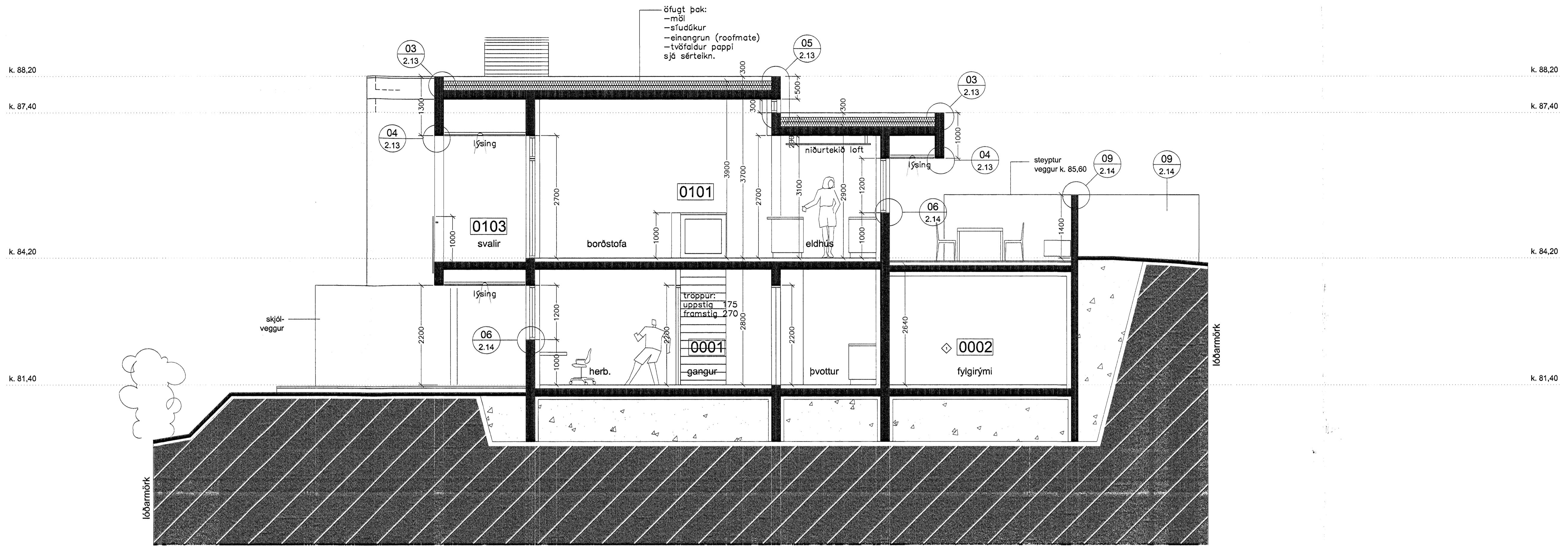
SNEIDING A - A M 1 : 50
