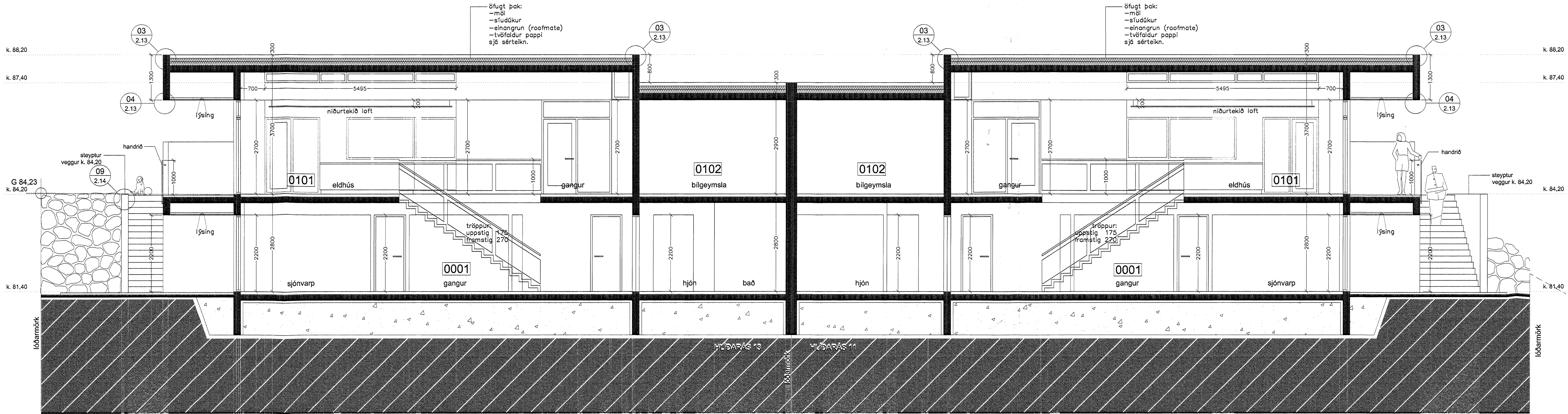
SNEIDING B - B M 1 : 50
