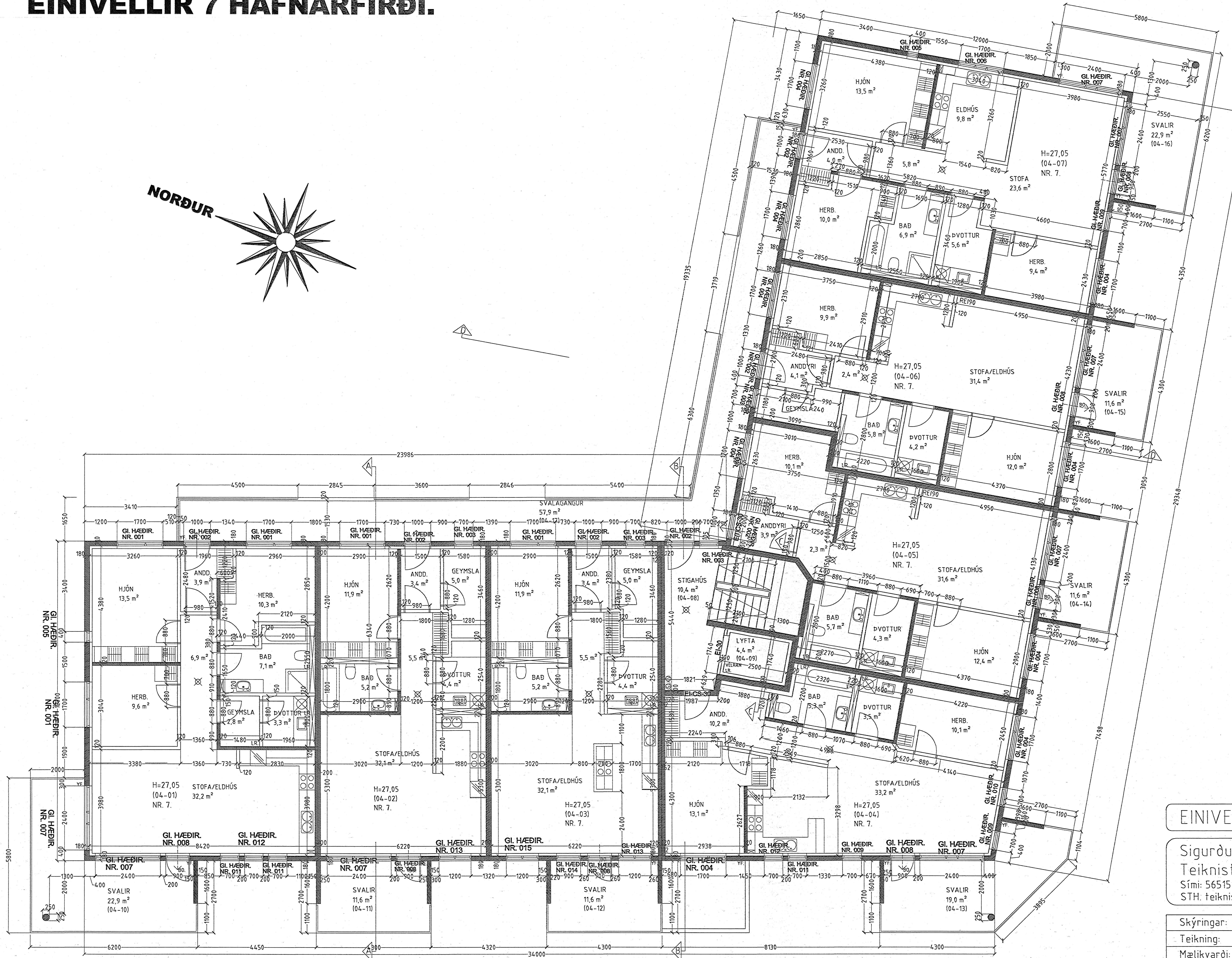
GRUNNMYND 4. HÆÐ MKV. 1:50.
