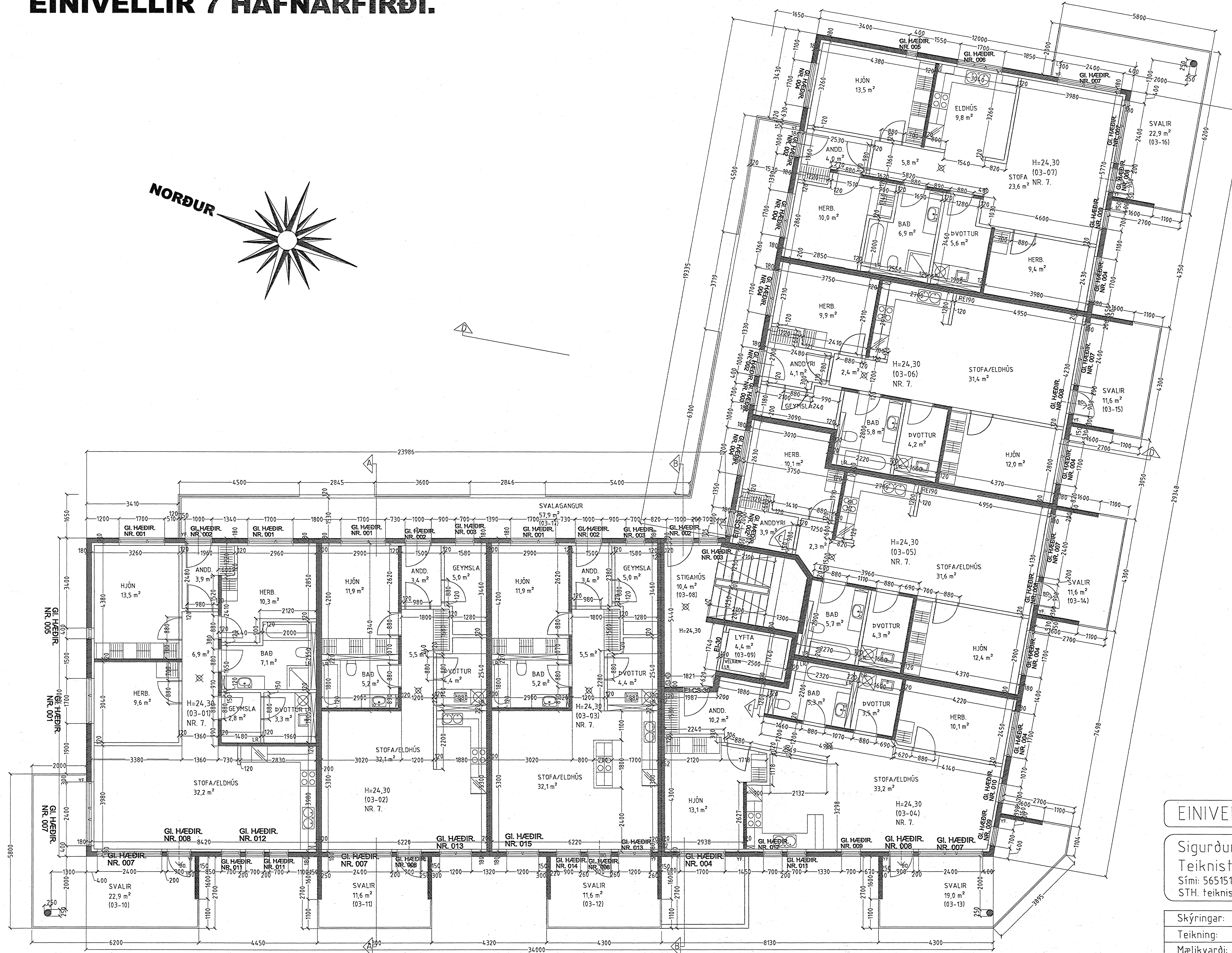
GRUNNMYND 3. HÆÐ MKV. 1:50.
