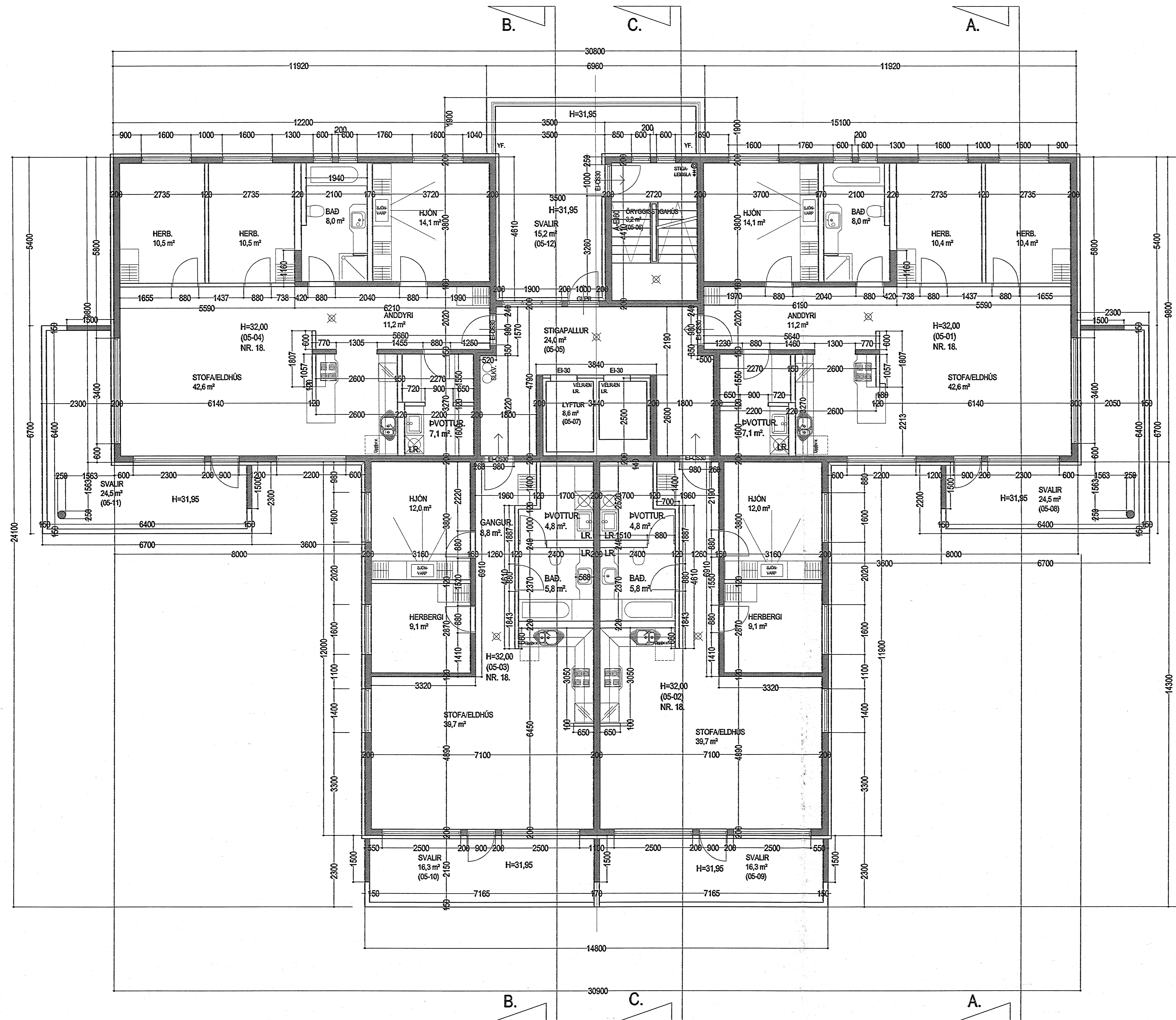
GRUNNMYND 5. HÆÐ MKV. 1:50.
