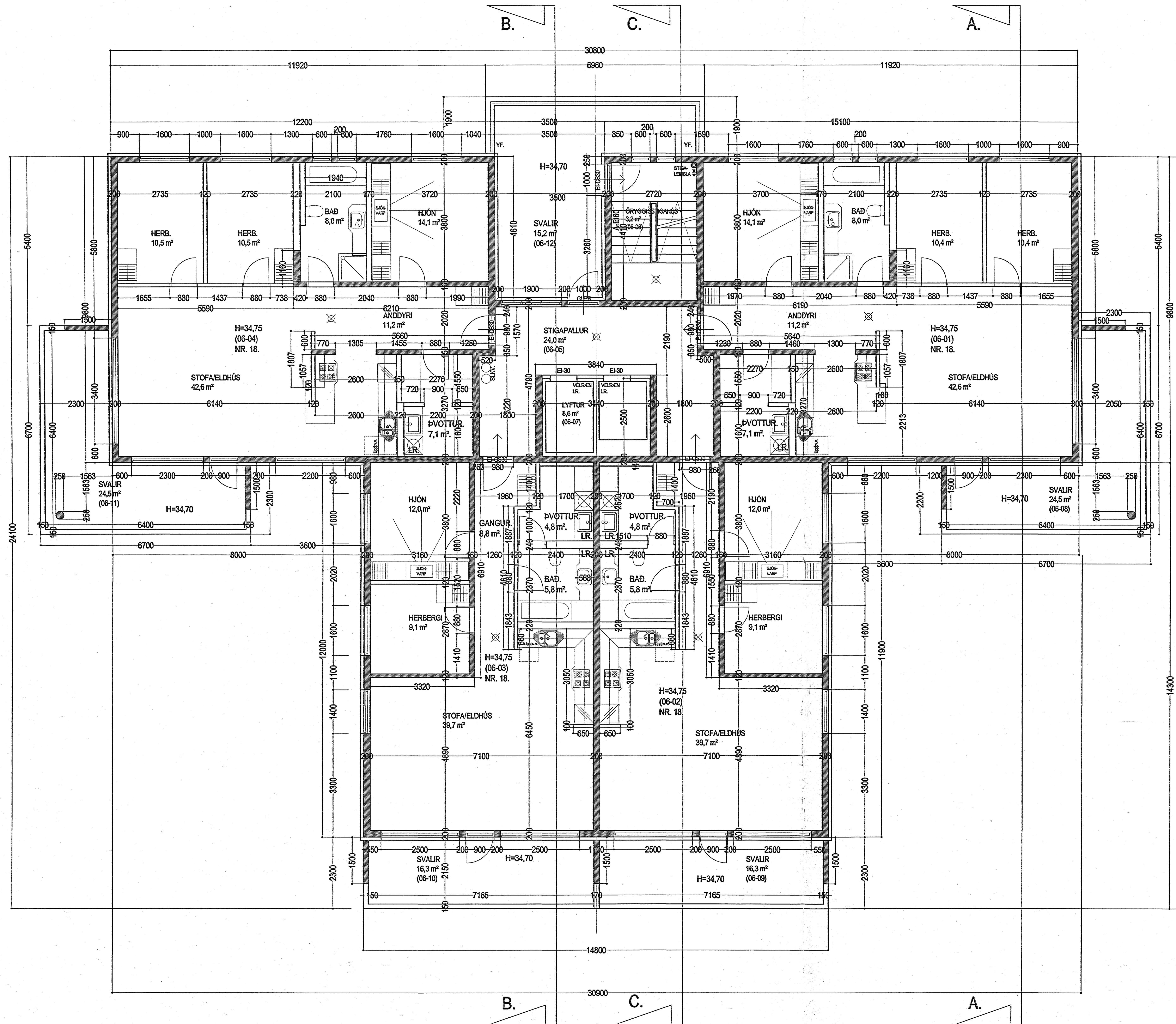
GRUNNMYND 6. HÆÐ MKV. 1:50.
