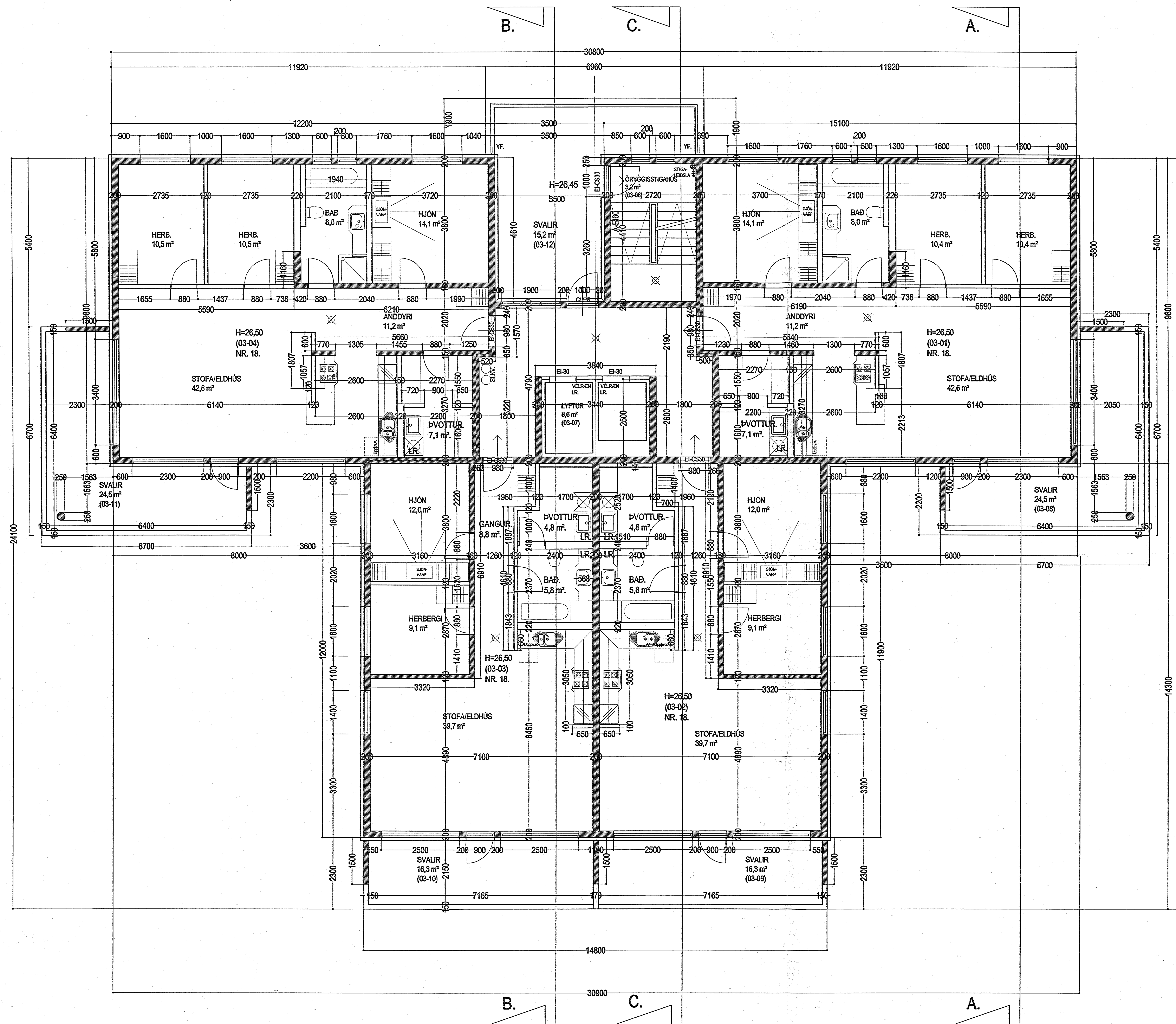
GRUNNMYND 3. HÆÐ MKV. 1:50.
