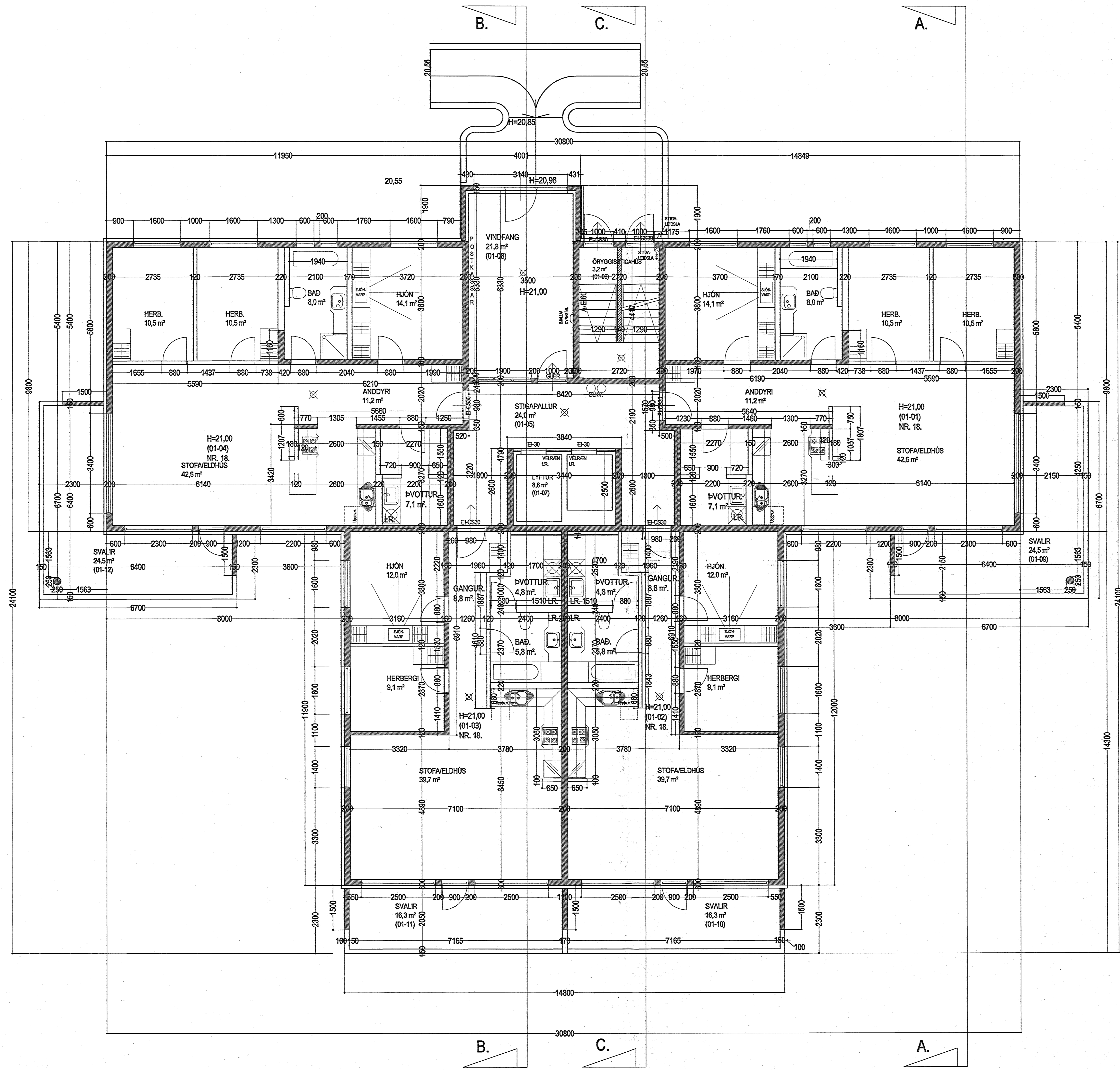
GRUNNMYND 1 HÆÐ. MKV. 1:50.
