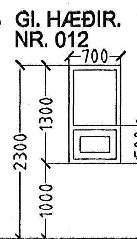
GI. HÆÐIR. NR. 012 10 stk. VESTUR
