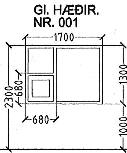
GI. HÆÐIR. NR. 001 20 STK AUSTUR. 5 STK NORÐUR.
