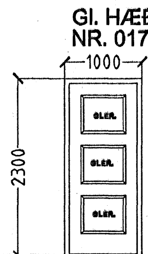
GI. HÆÐIR. NR. 017 ANDDYRI STOGAHÚSS. 1. STK HURÐ OPNAST HÆGRI INN.
