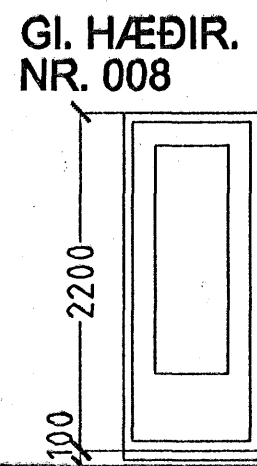
GI. HÆÐIR. NR. 008 SVALAHURÐIR. 15 stk opnist hægri út. 20 stk opnist vinstri út.
