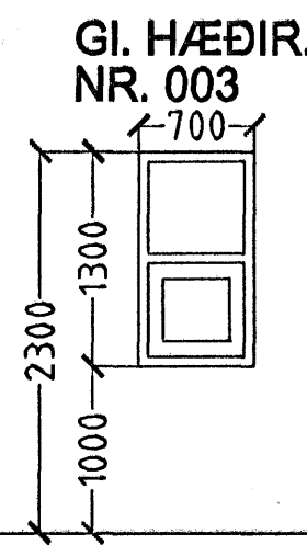
GI. HÆÐIR. NR. 003 5 stk. NORÐUR 15 stk AUSTUR
