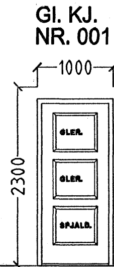
GI. KJ. NR. 001 Bítakjallari.. 1. STK HURÐ OPNAST VINSTRI ÚT..
