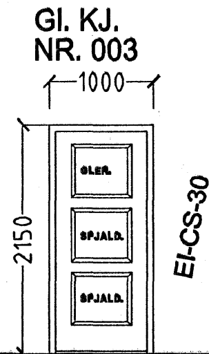
GI. KJ. NR. 003 BRUNASTÚKA.. 1. STK HURÐ OPNAST HÆGRI ÚT..
