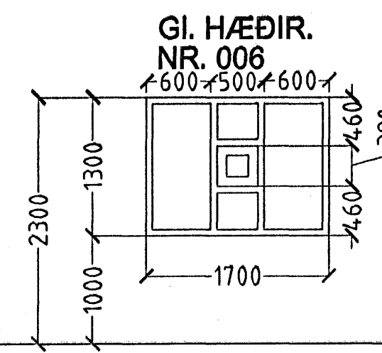
GI. HÆÐIR. NR. 006 5 stk. AUSTUR
