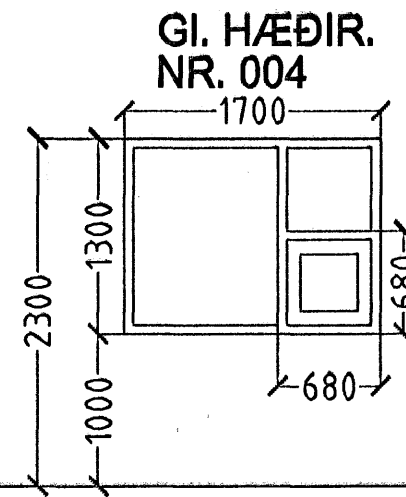
GI. HÆÐIR. NR. 004 20 stk. NORÐUR 20 stk. SUÐUR 4 STK VESTUR
