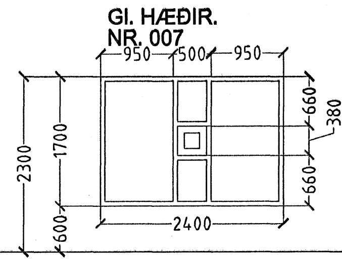
GI. HÆÐIR. NR. 007 5 stk. NORÐUR 15 stk. SUÐUR 5 stk AUSTUR. 15 stk VESTUR.
