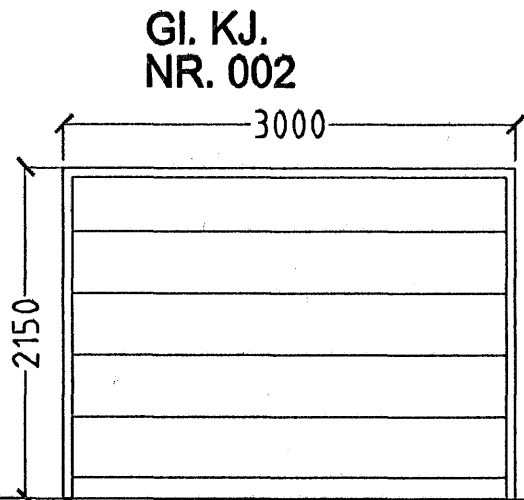
GI. KJ. NR. 002 1. STK. BÍLAKJALLARI.
