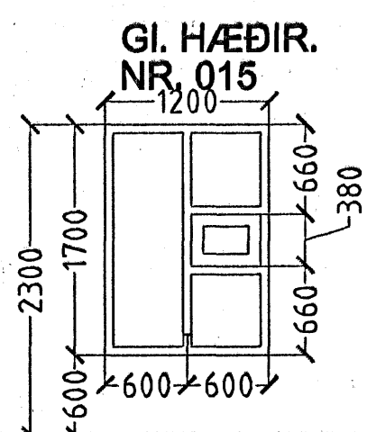
GI. HÆÐIR. NR. 015 5 stk. VESTUR
