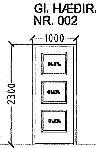
GI. HÆÐIR. NR. 002 ANDDYRISHURÐIR/ STIGAHÚS. 25 stk opnist inn Vinstri 5 stk opnist inn Hægri 5 STK opnist INN VINSTRI EI(I)CS 30.
