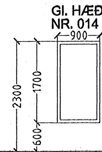
GI. HÆÐIR. NR. 014 5 stk. SUÐUR
