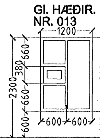
GI. HÆÐIR. NR. 013 10 stk. SUÐUR
