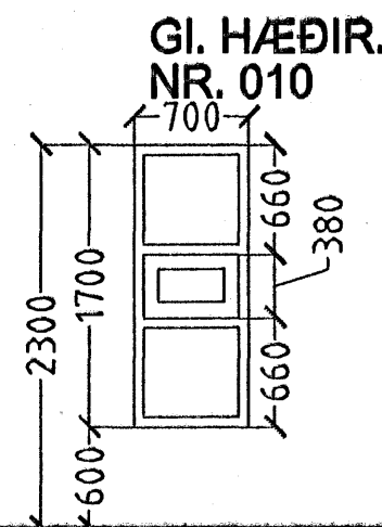
GI. HÆÐIR. NR. 010 5 stk. SUÐUR
