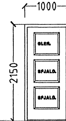
GI. KJ. NR. 006 HJÓL OG VAGNAR.. 1. STK HURÐ OPNAST VINSTRI INN.
