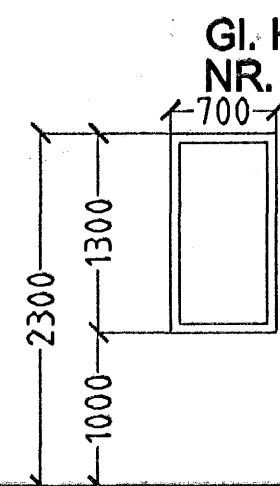
GI. HÆÐIR. NR. 011 15 stk. VESTUR
