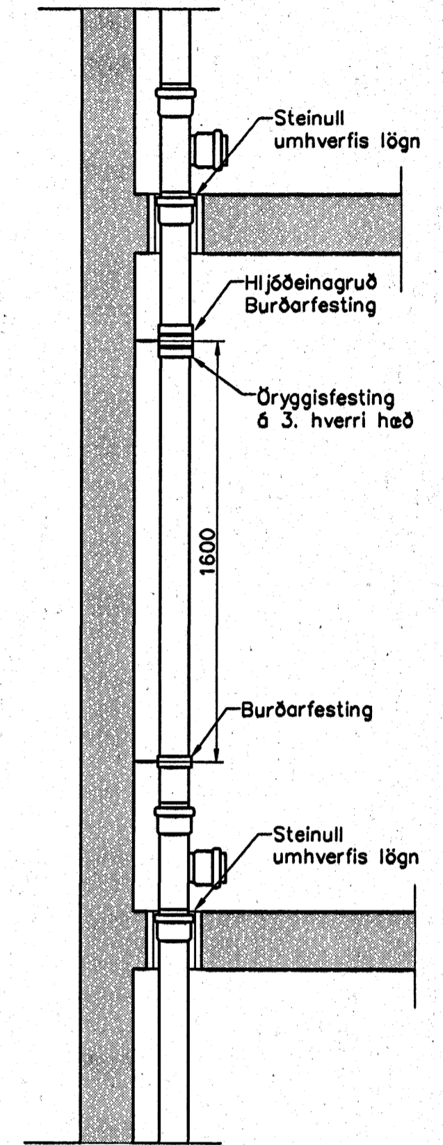
Fallpípa, festingar 1:20
