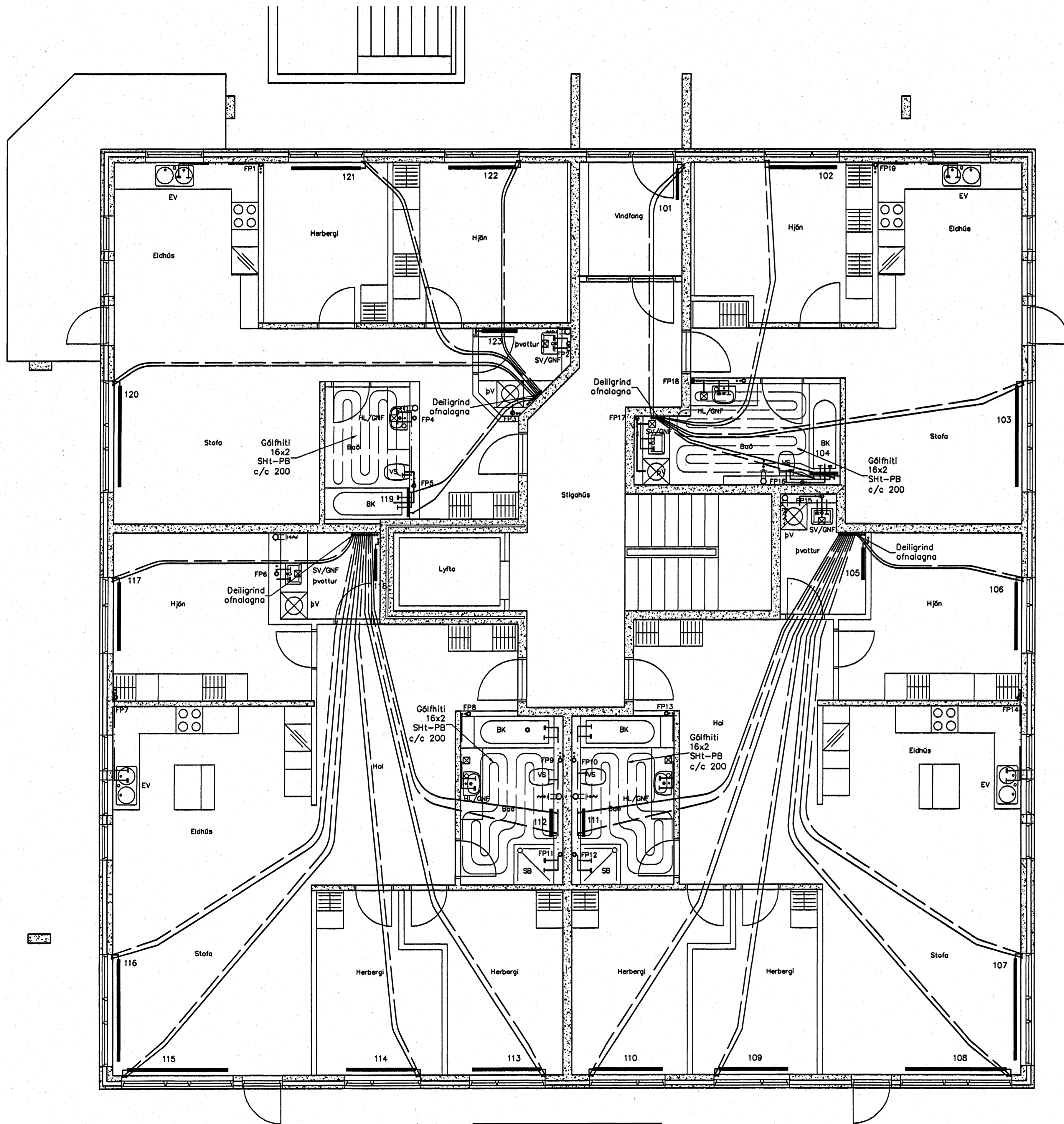
Lagnir 1. hæð, Grunnmynd, 1:50
