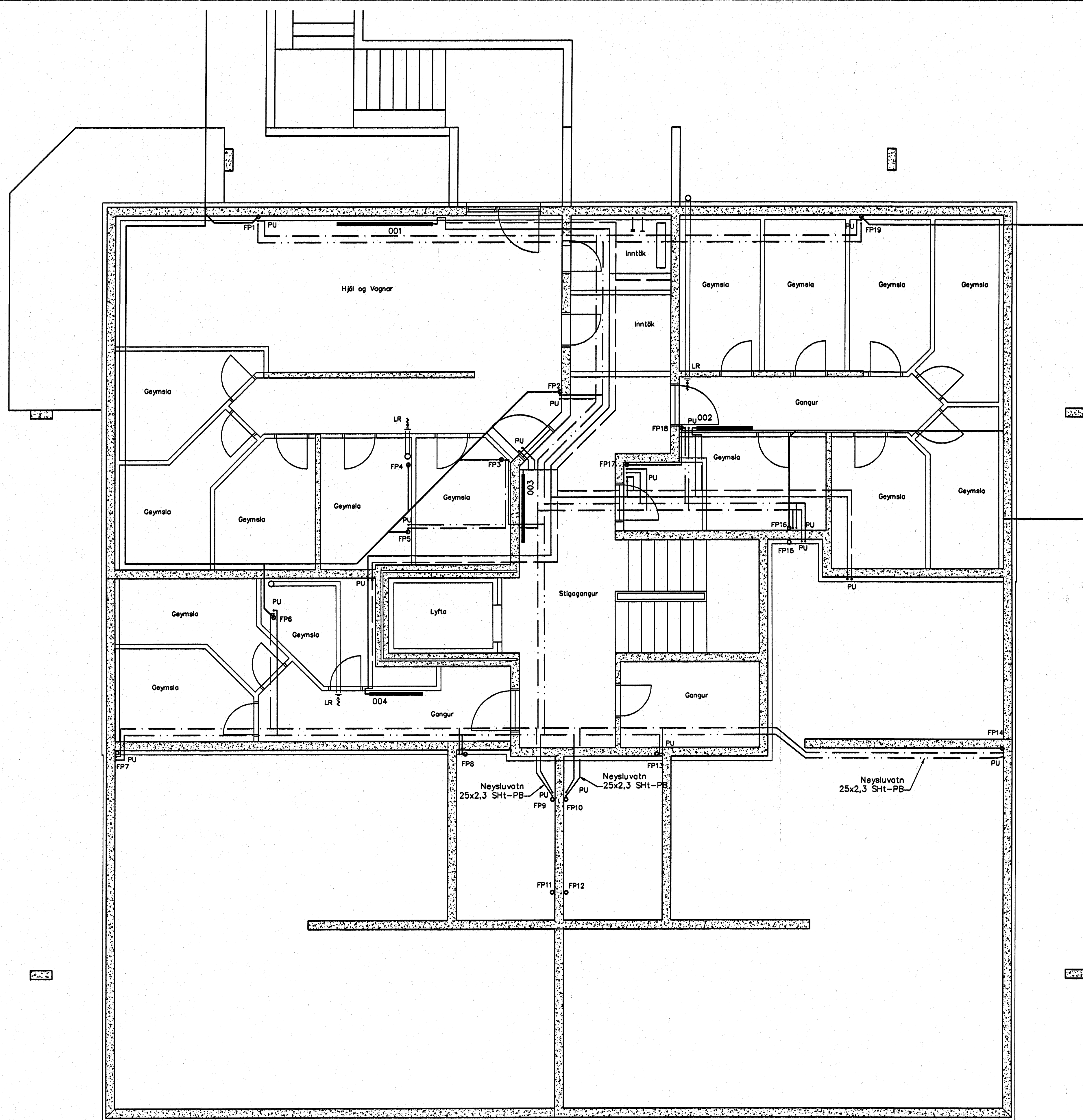
Lagnir kjallara, Grunnmynd, 1:50
