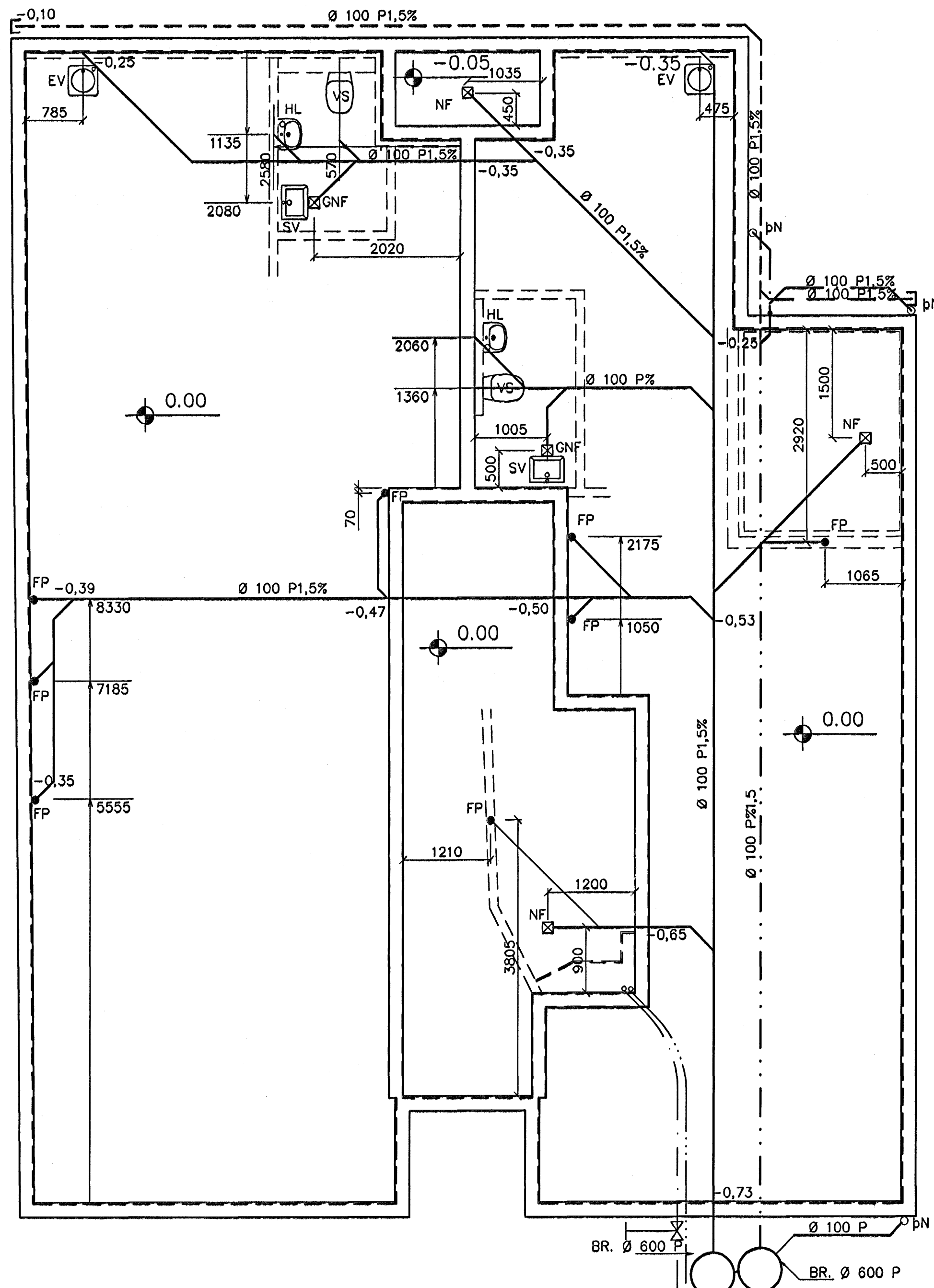
GRUNNMYND 1:50
