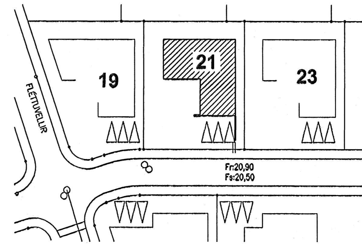
Afstöðumynd 1:500
