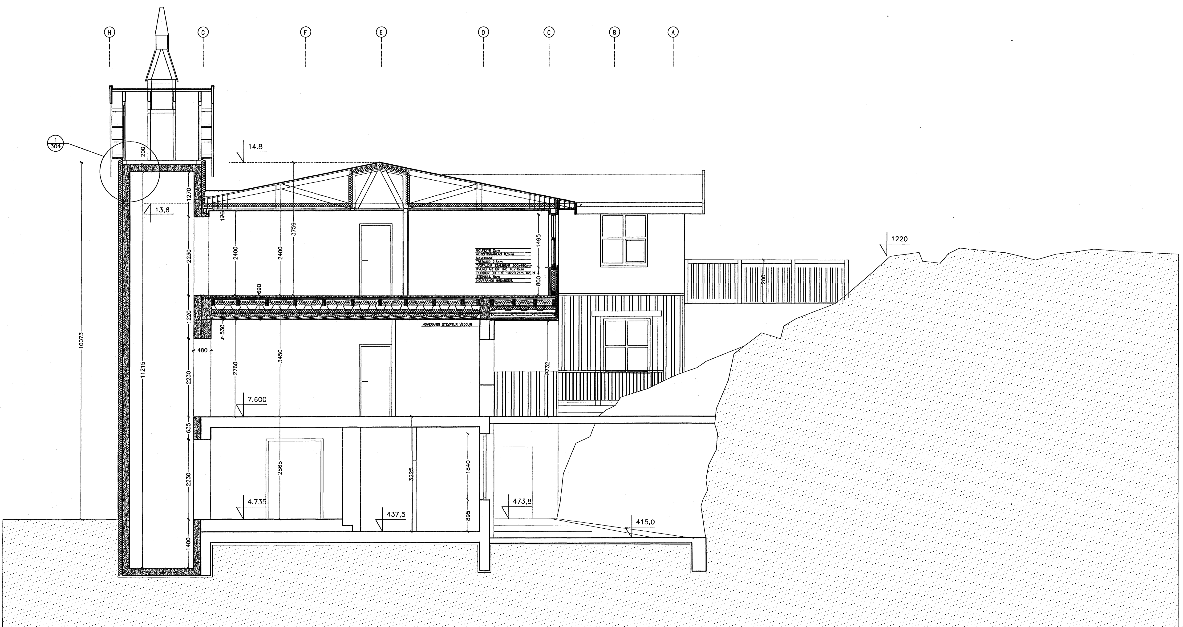
SNID B-B 1:50
