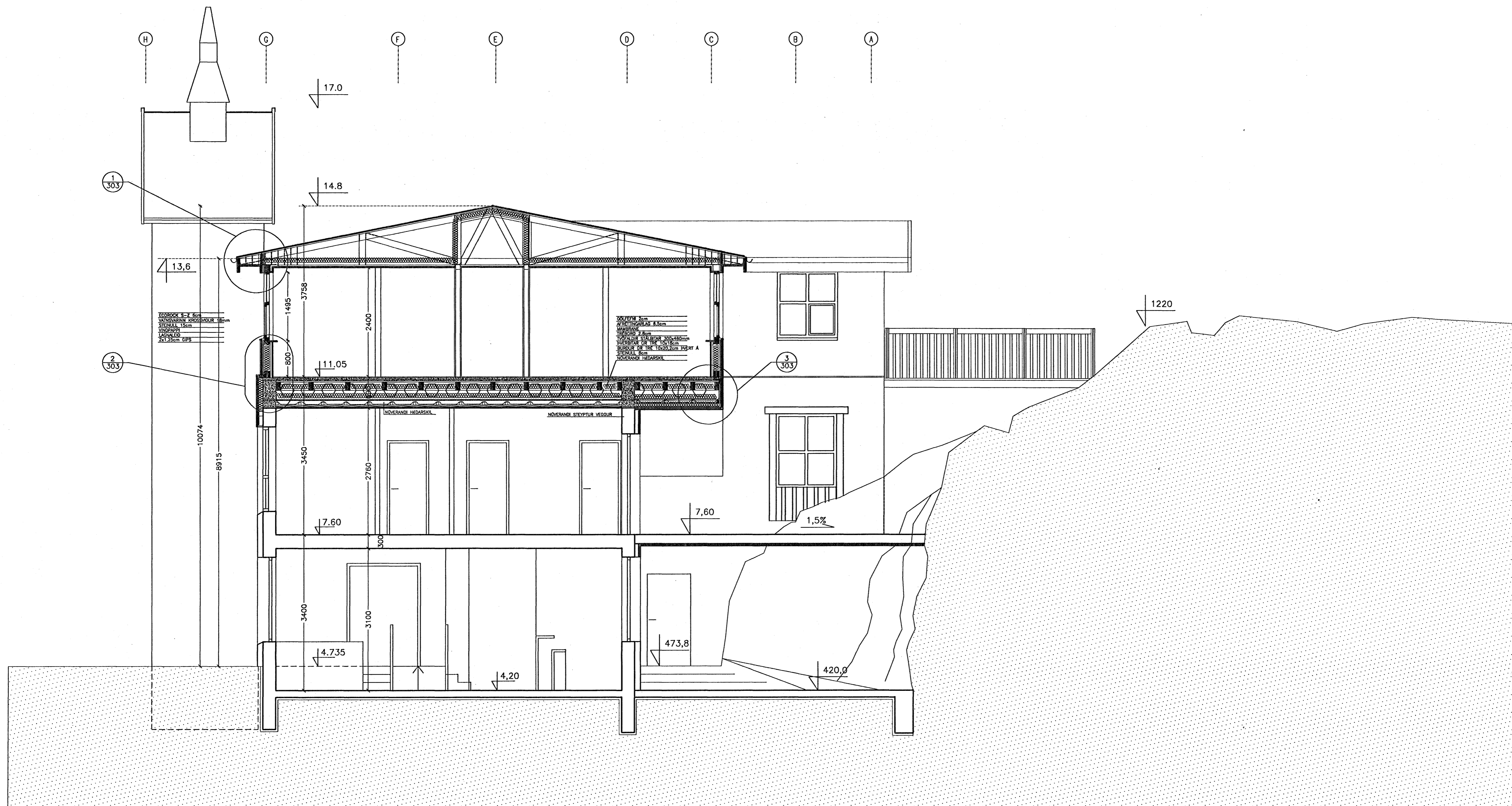
SNID A-A 1:50
