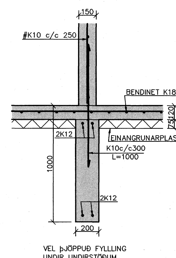
DEILL 1:20 F B02
