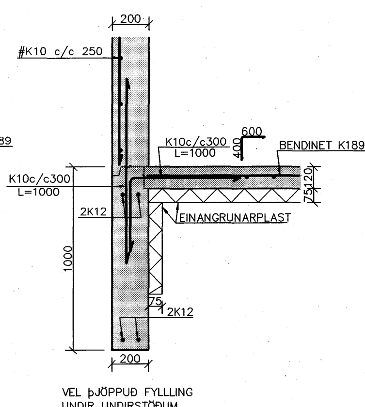
DEILL 1:20 C B02
