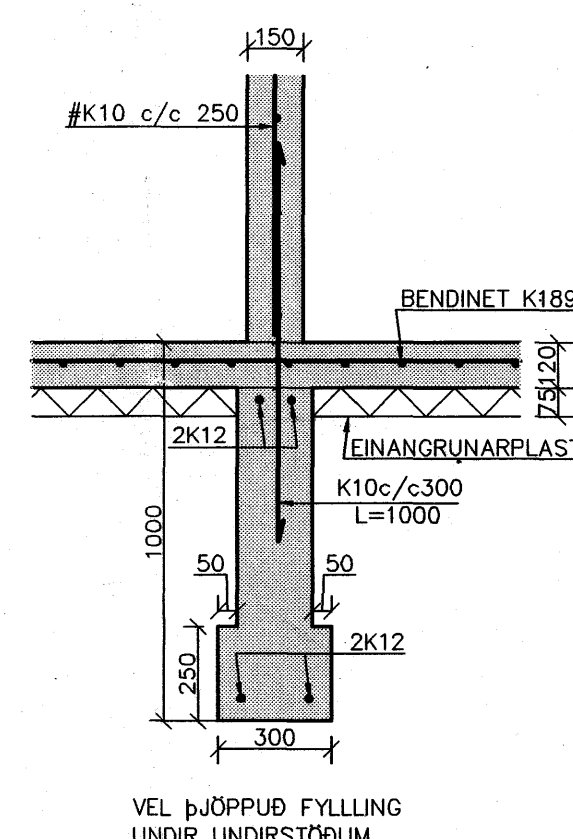
DEILL 1:20 E B02
