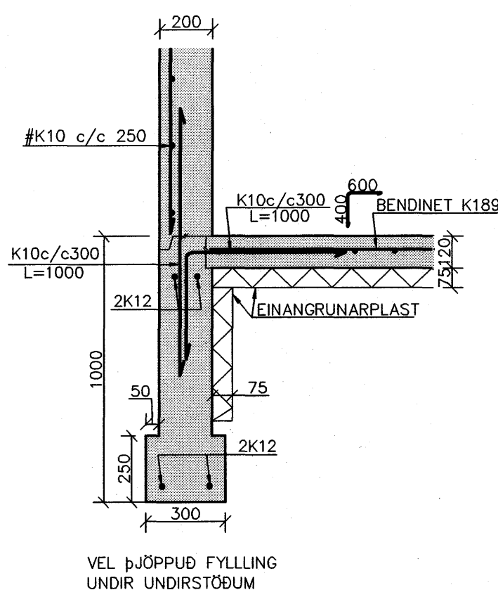
DEILL 1:20 A B02
