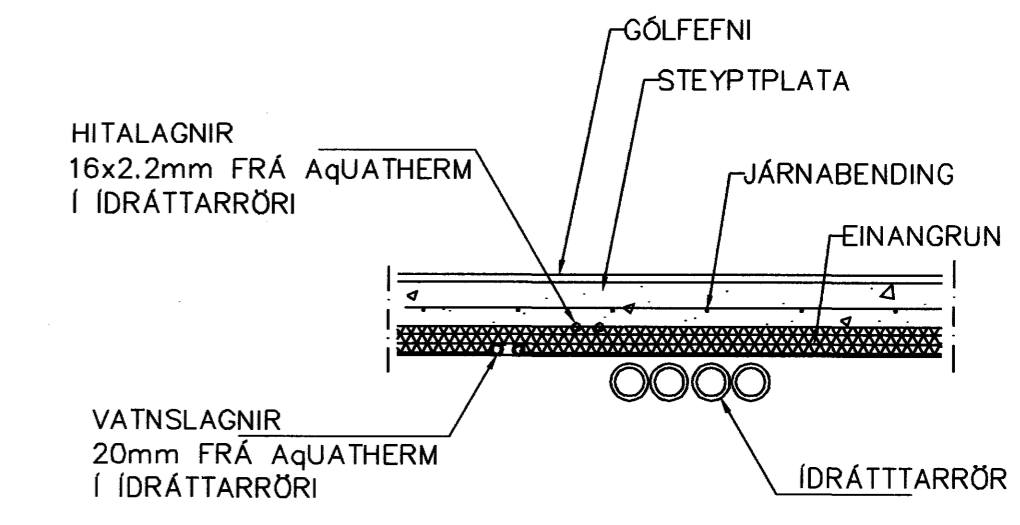
LAGNIR, SNIÐ, 1:20
