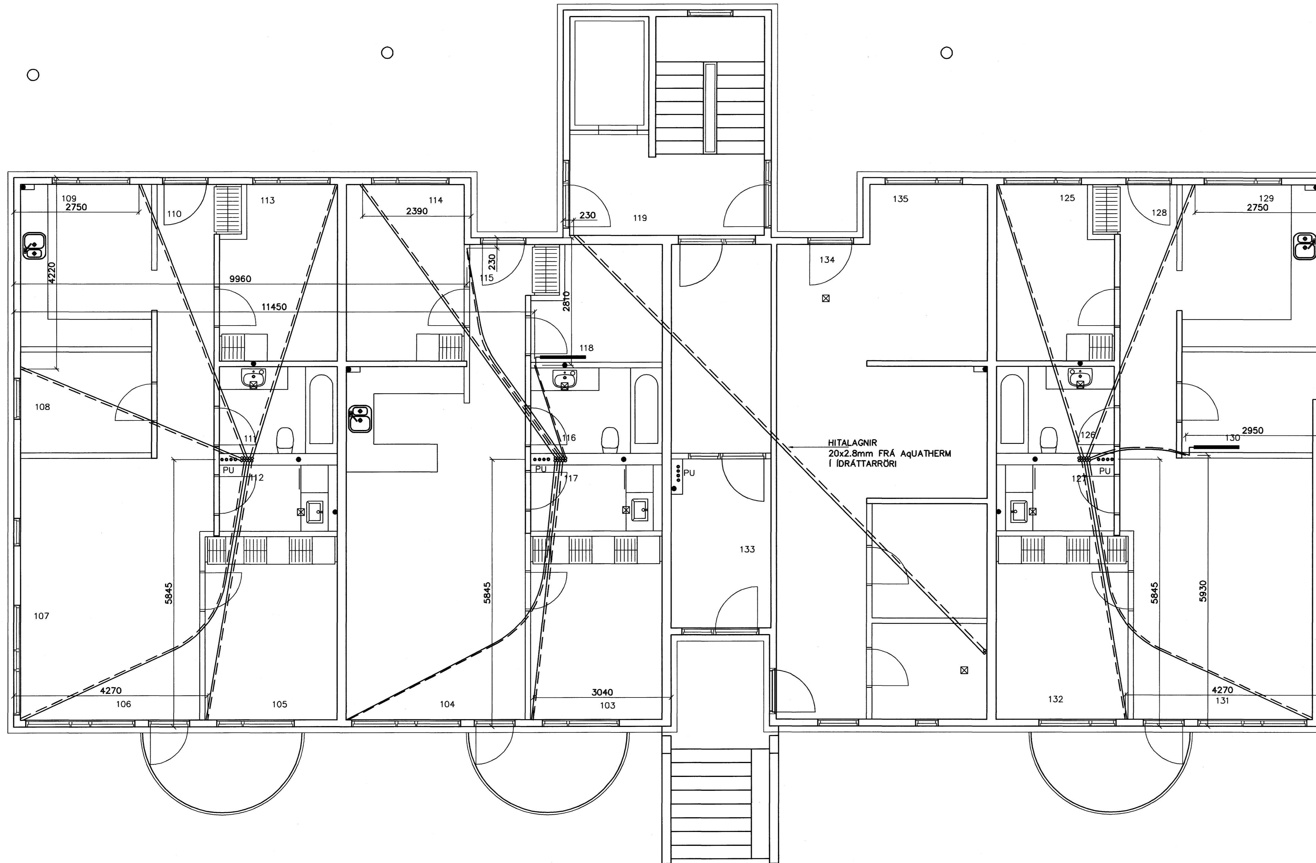
GRUNNMYND 1 HÆÐAR 1:50
