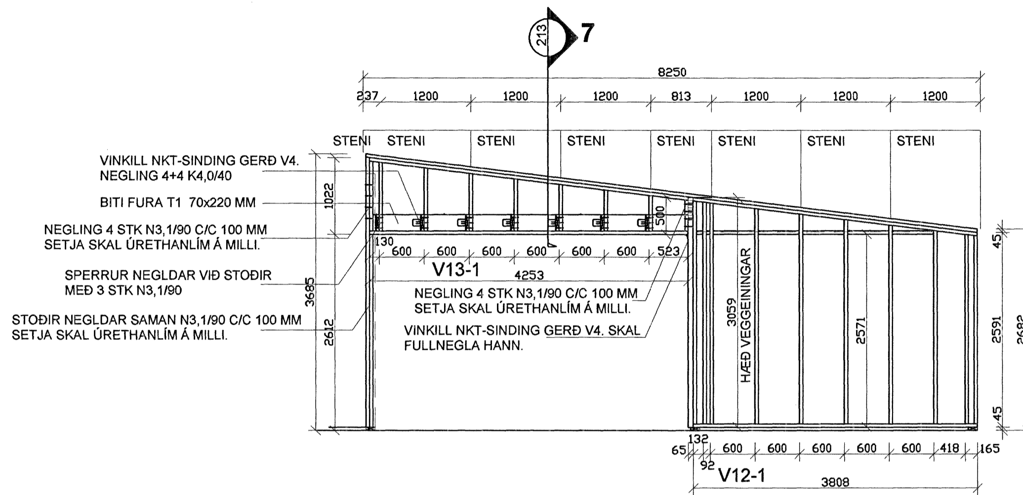
V12 OG V13 ÚTLIT - 1:50
