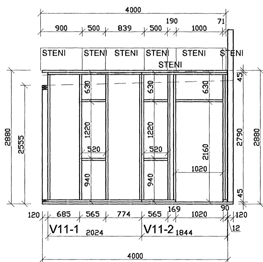
V11 ÚTLIT - 1:50
