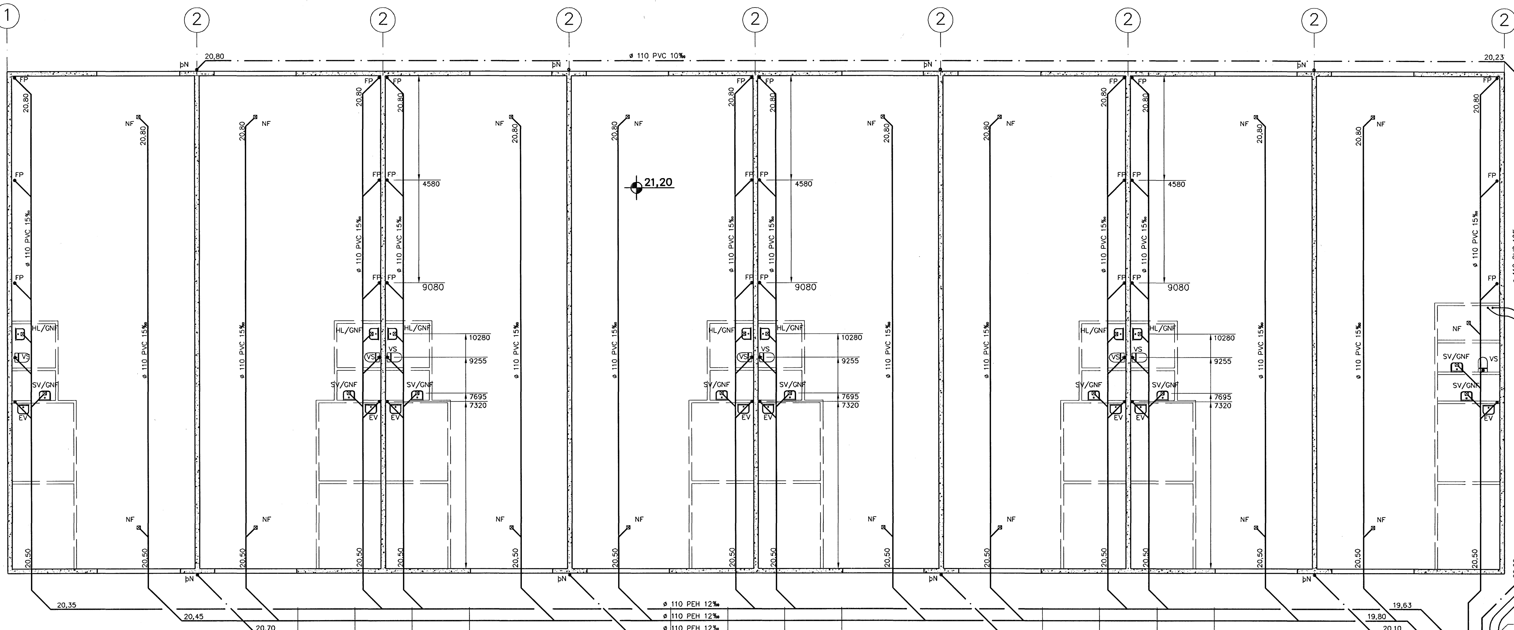
Grunnlagnir, Grunnmynd, 1:100
