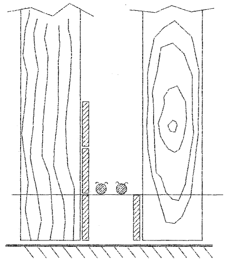
SNÍÐ A - A Í SÖKKULVEGG SÝND ERU 2 NEDSTU STEYPU-STYRKJARJÁRN Í STEYPUÓTI OFAN Á NEDSTU MÓTAVIRUM
