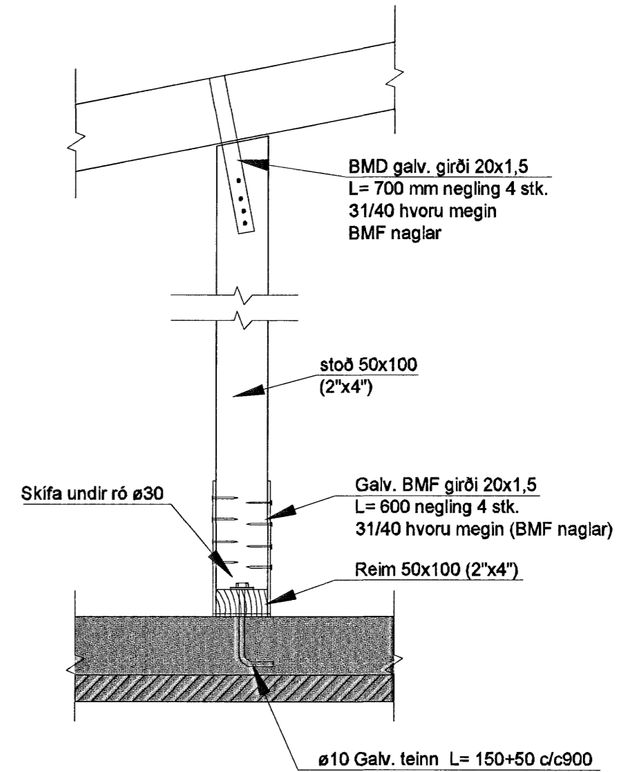
A-114 SNIÐ. 1:10
