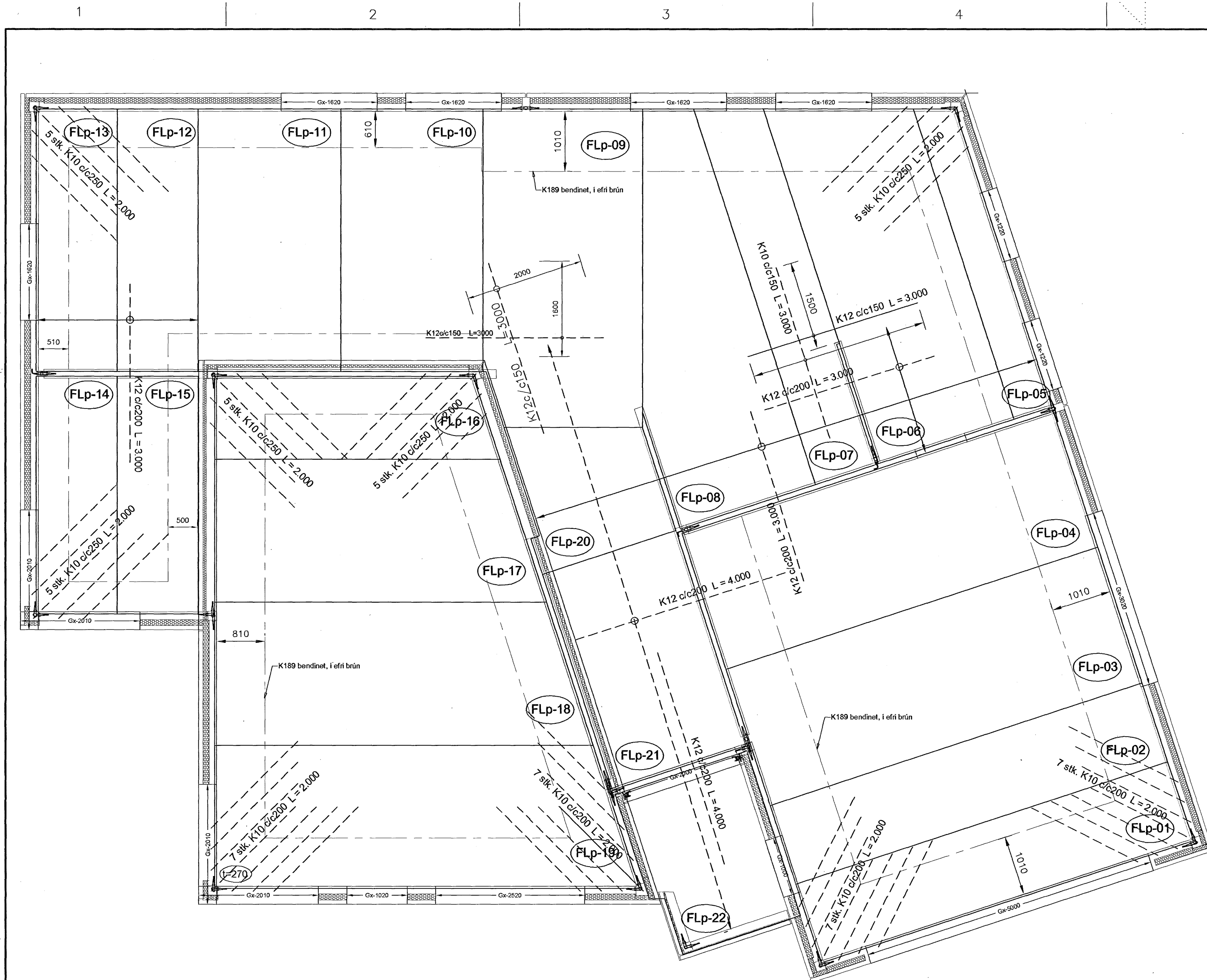
GRUNNMYND - LOFTAPLÖTUR, EFRI JÁRNBENDING 1:50
