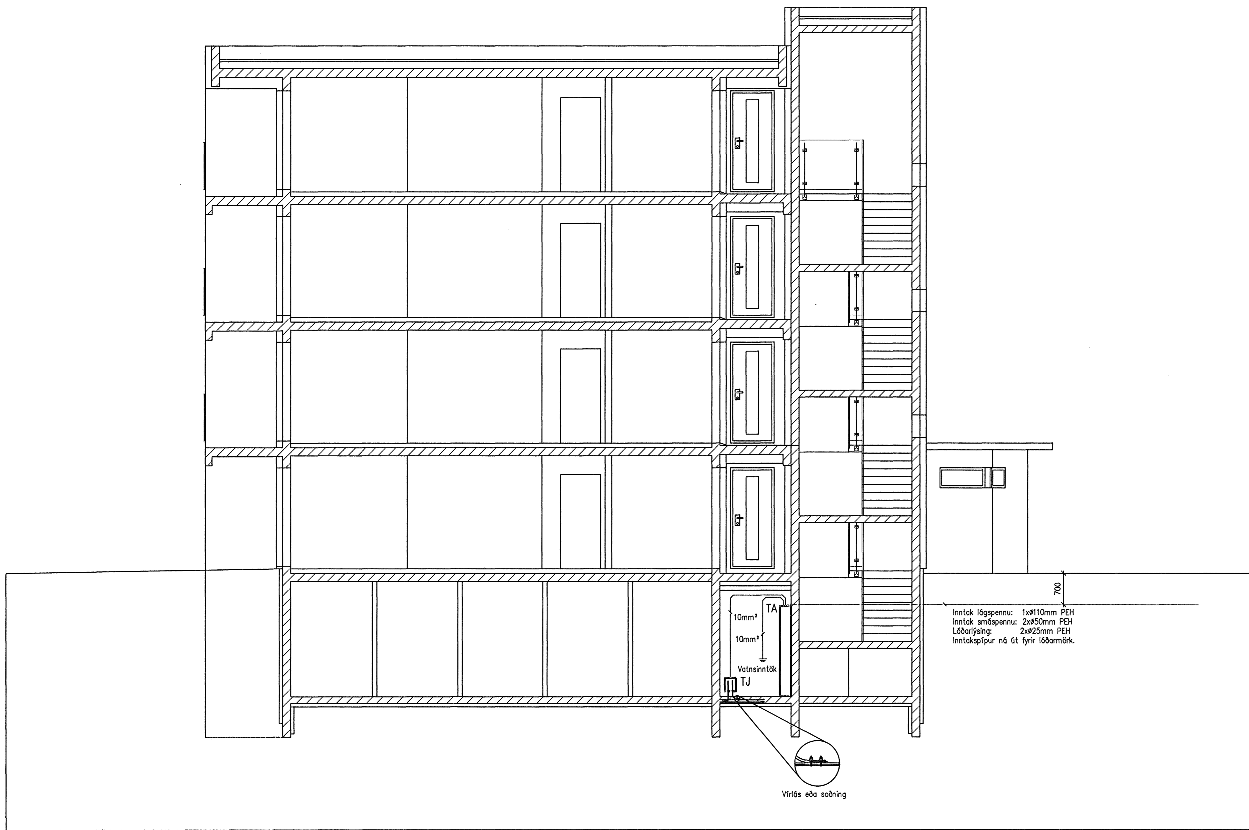
Snið A-A 1:50
