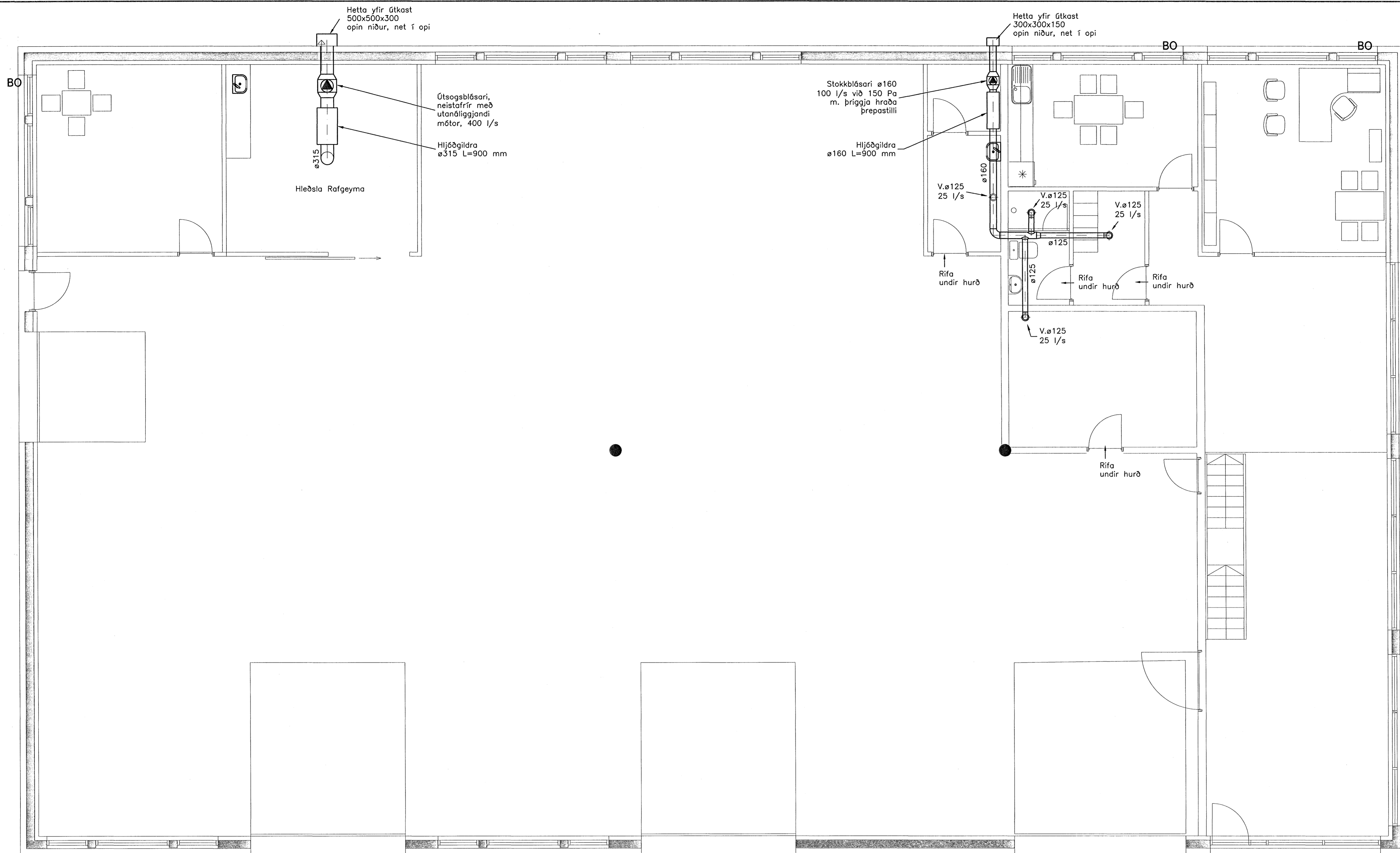
A Grunnmynd - Loftþræsing - 1. hæð L-001 1:50
