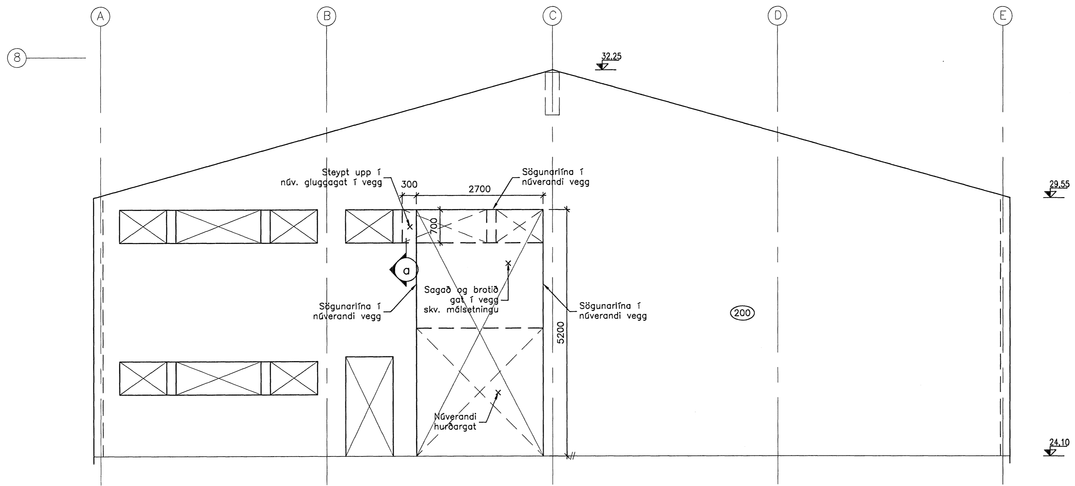
V4 HLIÐARMYND – SÖGUN OG BROT ÚR NÚVERANDI VEGG - 1:50
