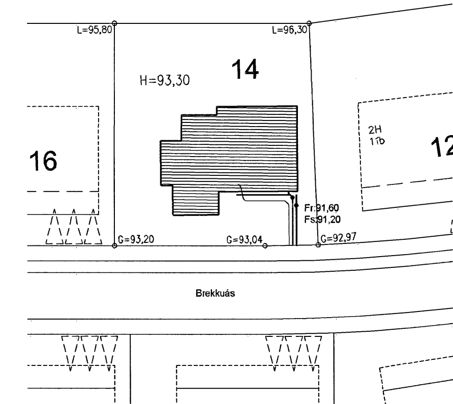
Afstöðumynd 1:500
