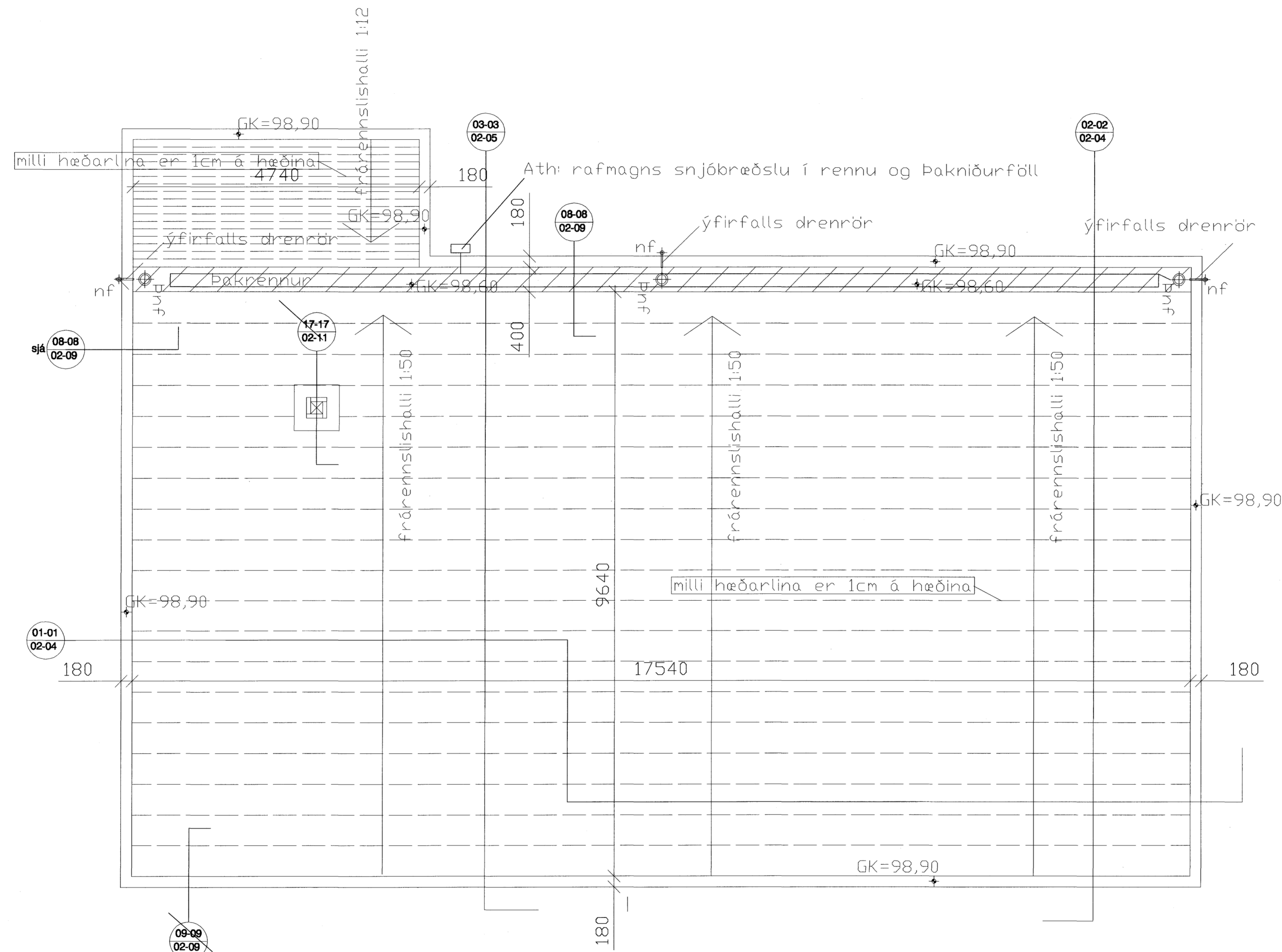
Þakmynd.(hæðarlega Þaks)
