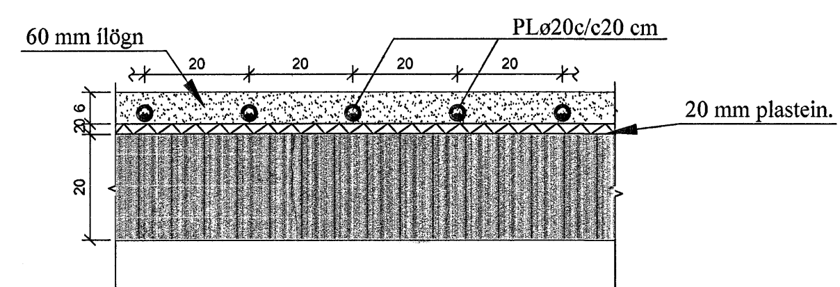
SNIÐ X - X. 1:10
