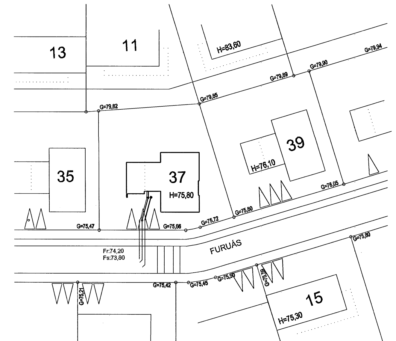
Afstöðumynd 1:500
